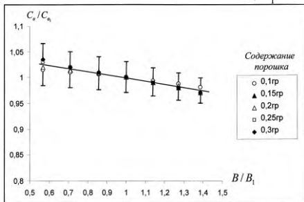
Рис.4. Зависимость относительной теплоемкости C_a/C_{a_1} от относительного магнитного поля B/B_1
