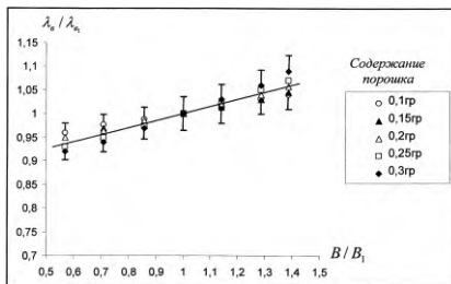
Рис.3. Зависимость относительной теплопроводности \lambda_a/\lambda_{a_1} от относительного магнитного поля B/B_1
