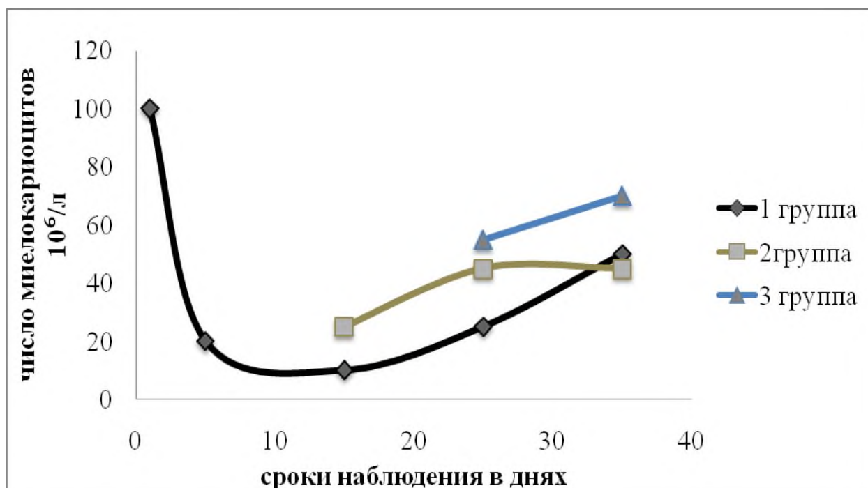
Рис. 5. Влияние фитοэкстракта из Chondrilla Laticoronata Leonova на темпы прироста миелокариоцитов при фракционированном х-облучении
