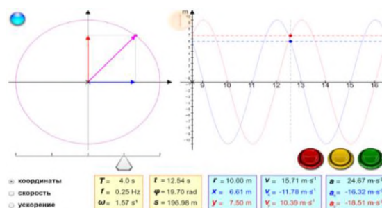
Рис. 2.2 Движение тела по окружности
