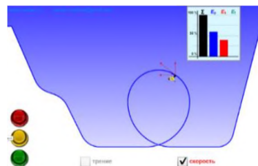
Рис. 2.3 Закон превращения и сохранения энергии.
