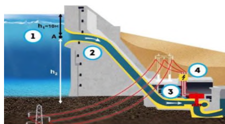
Рис. 2.4 Схематический вид ГЭС.
