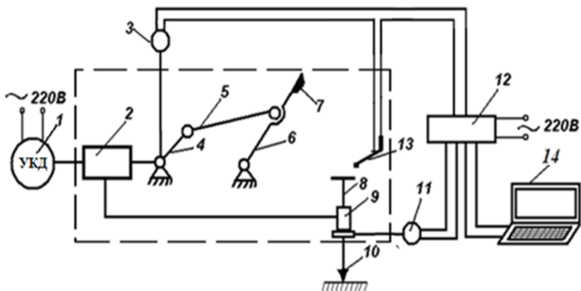
Рисунок 4.18 - Экспериментальный стенд
