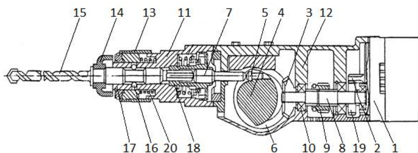
Рисунок 1.12 – Конструкция электромеханического перфоратора ПРЭ – 1
