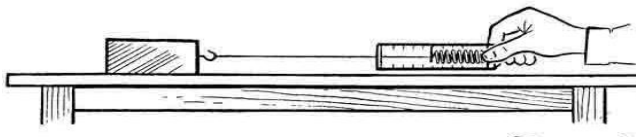
Рис.4. Определение коэффициента трения
