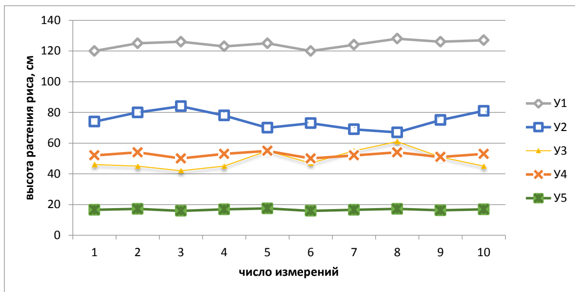
Рисунок 3 - Диаграммы измерения высота растения риса (сорт Ак-урук): Y_1 = X + 124,2 -высота растения риса до уборки, см; Y_2 = X + 76,1 -высота растения риса после уборки, см; Y_3 = X + 49,18 -высота растения риса оставшийся на почве, см; Y_4 = X + 52,4 -длина окружности снопов растения риса, см; Y_5 = X + 16,72 ; -диаметры снопов растения риса, см.
