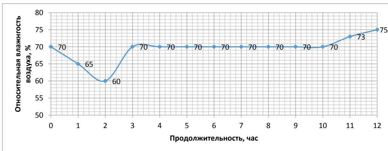
Рисунок 8. 55 – градусный режим паро-термической обработки.
