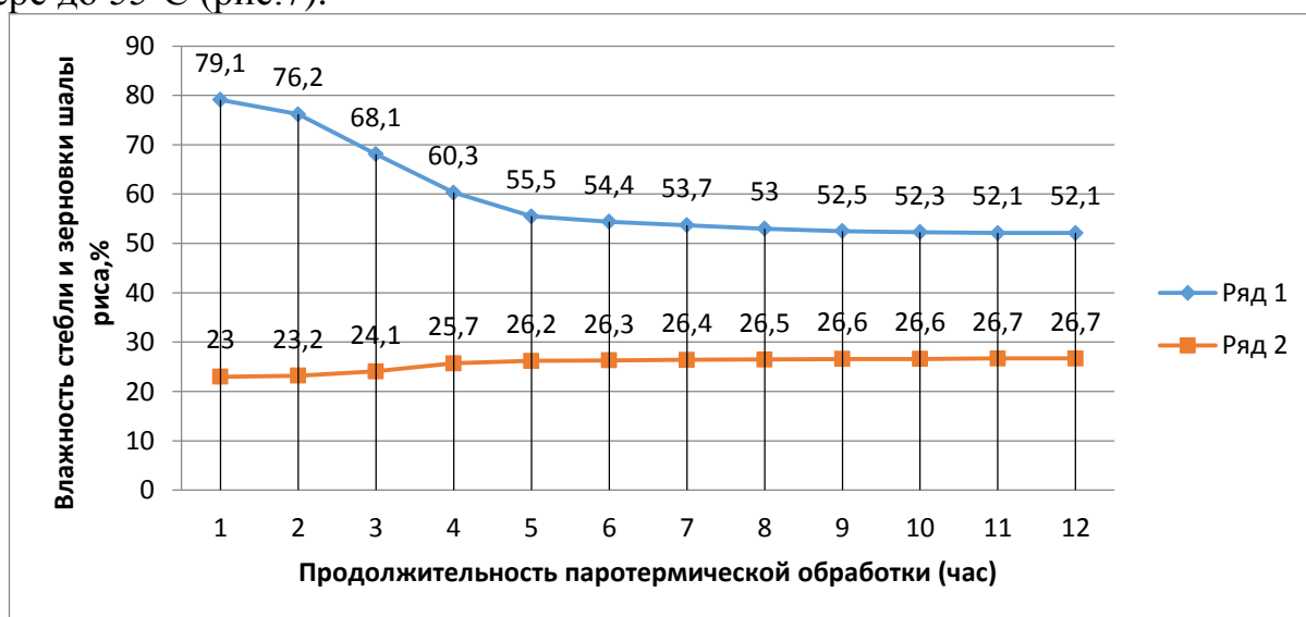
Рисунок 7 - Диаграмма изменения влажности стебля и зерновки шалы растения риса от продолжительности паро-термической обработке на установке (t = 55°С, относительная влажность воздуха W = 65-70 %)
