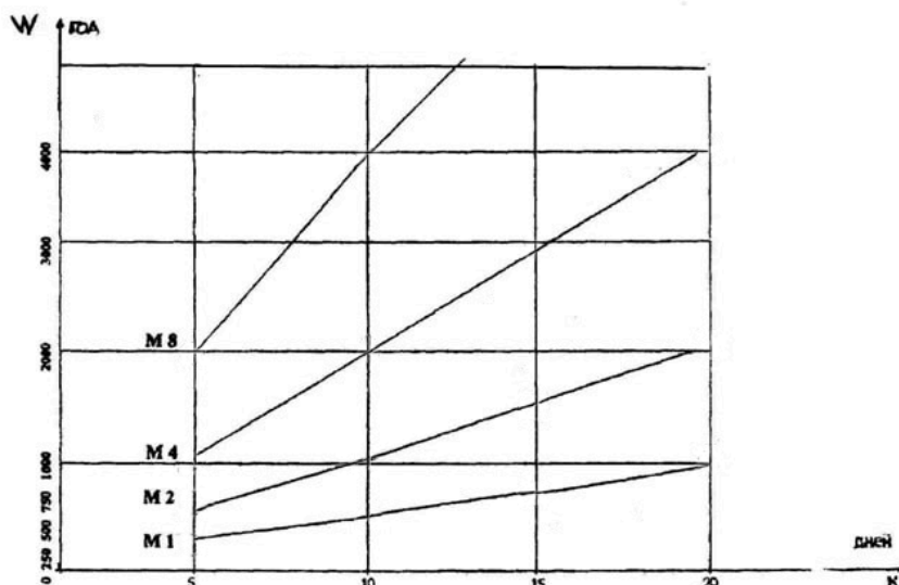
14-сүрөт. Кыркуучулардын өндүрүмдүүлүгүнүн (W) алардын санына (M) жана кыркуунун узактыгына (K) көз карандылыгы.
