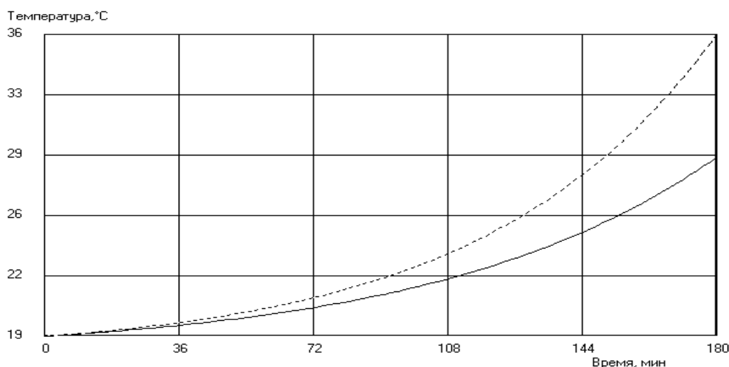
9-сүрөт. Ваннадагы жумушчу суюктуктун температурасынын ваннанын узактыгына жараша өзгөрүү графиги: — 1 — койлордун саны, 7ге барабар ; ..... 2 – койлордун саны 9га барабар.
