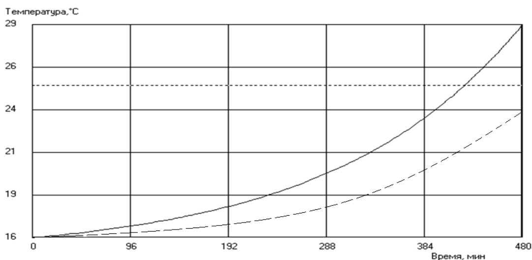
10-сүрөт. Койлорду жуунтуу үчүн ваннадагы суюктуктун көлөмүн эсепке алып, температуранын убакыттын өтүшү менен өзгөрүү графиги: — 1-суюктуктун температурасынын убакыттын өтүшү менен өзгөрүшүнүн ийри сызыгы ( V = 5000 литр); - - - 2 -суюктуктун температурасынын убакыттын өтүшү менен өзгөрүшүнүн ийри сызыгы ( V = 6000 литр); ..... 3 - уруксат берилген температуранын мааниси.
