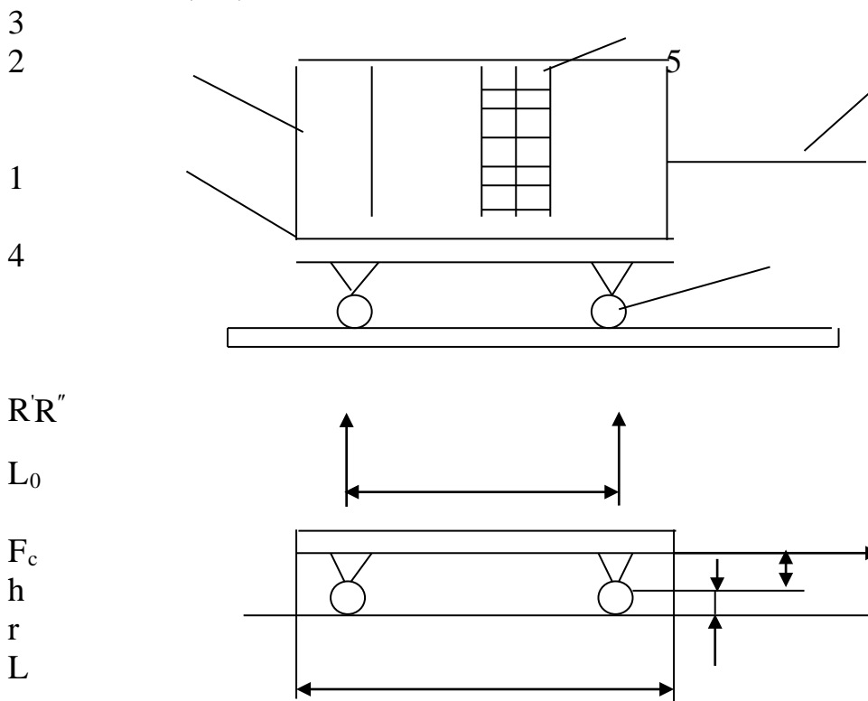
7 – сүрөт. Платформага аракеттенүүчү күчтөрдүн схемасы
