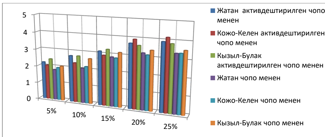
6-сүрөт – ККОнун бекемдигинин R активдештирилген жана активдештирилбеген бентонит чопосунун концентрациясынан көз карандылыгы
