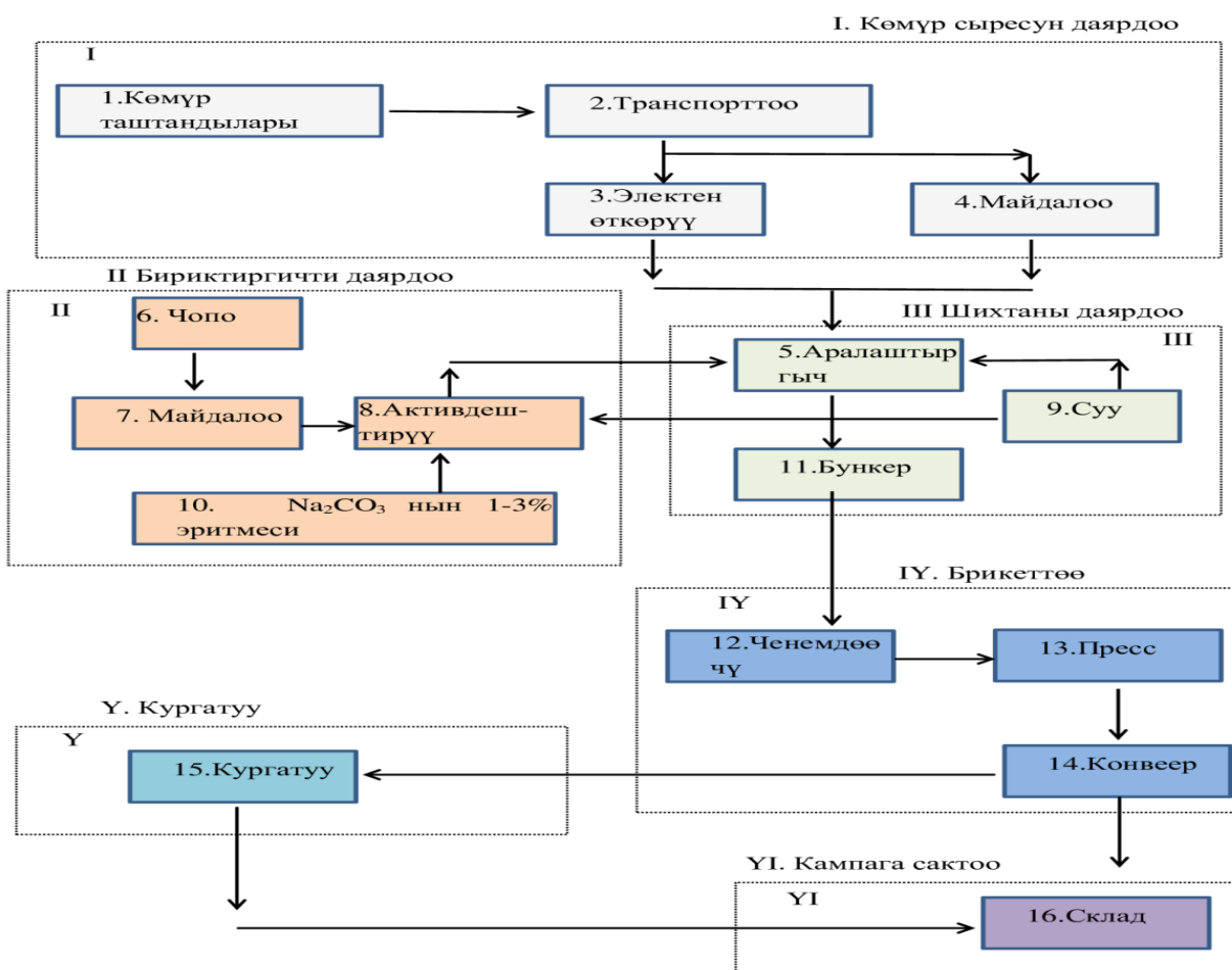
10-сүрөт – Бентонит жана лесс чополору менен көмүрдү брикеттөөнүн өнөр жай технологиясынын технологиялык схемасы
