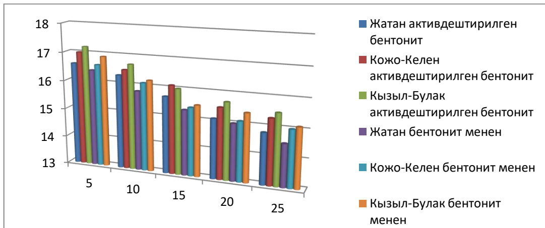
7-сүрөт – ККОнун Q калориялуулугунун активдештирилген жана активдештирилбеген бентониттин концентрациясынан көз карандылыгы
