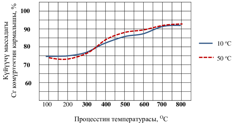
2-сүрөт – Жатан көмүрүнүн ар түрдүү ылдамдыкта ысытууда катуу калдыктардагы көмүртектин салмактык процентте кармалышы
