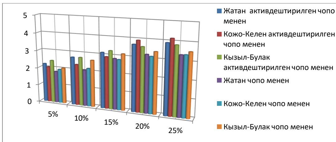
6-сүрөт – ККОнун бекемдигинин Р активдештирилген жана активдештирилбеген бентонит чопосунун концентрациясынан көз карандылыгы
