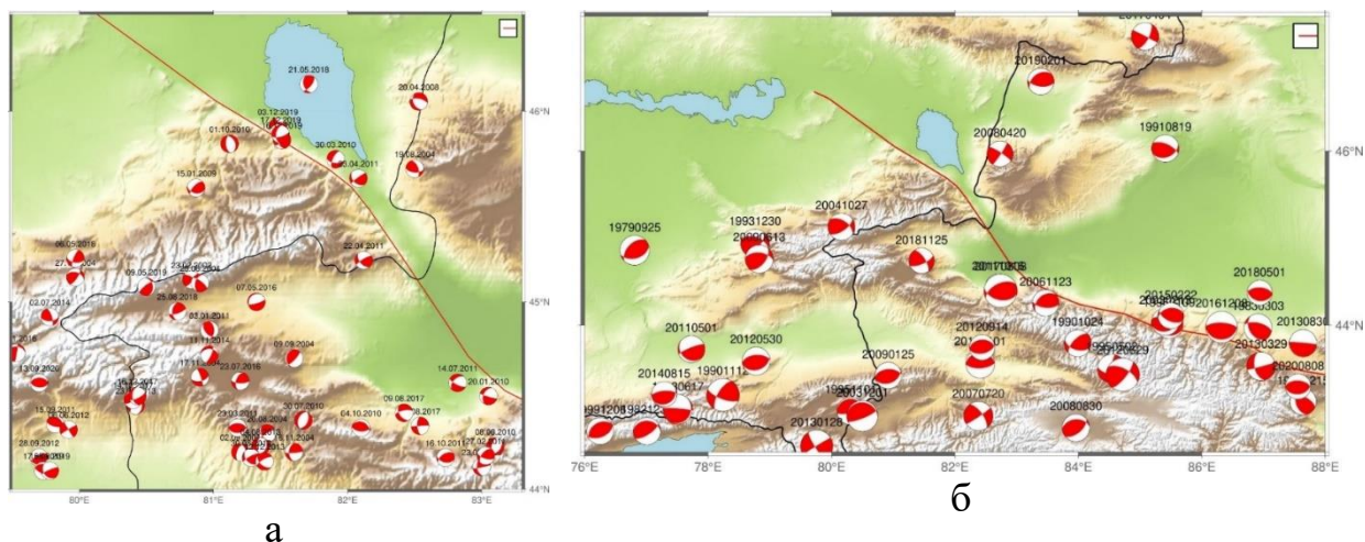
Рисунок 2.6. Карта механизмов очагов землетрясений Джунгаро-Северо-Тянь-Шаньского региона (а) по данным каталогов COME и ИГИ, (б) по данным каталога GCMT.
