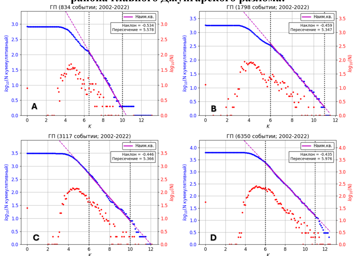
Рисунок 2.5. График повторяемости землетрясений района главного Джунгарского разлома. Сегменты А, В, С, D за 2002-2022гг.
