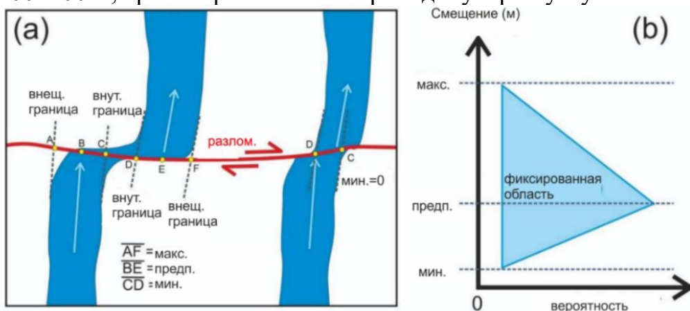
Рисунок 2.7. Измерение бокового смещения по руслам водотоков с использованием спутниковых изображений. (а) и иллюстрация того, как
