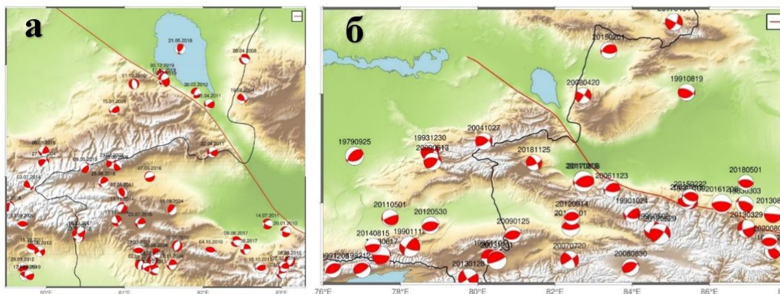
Рисунок 2.6. Карта механизмов очагов землетрясений Джунгаро-Северо-
