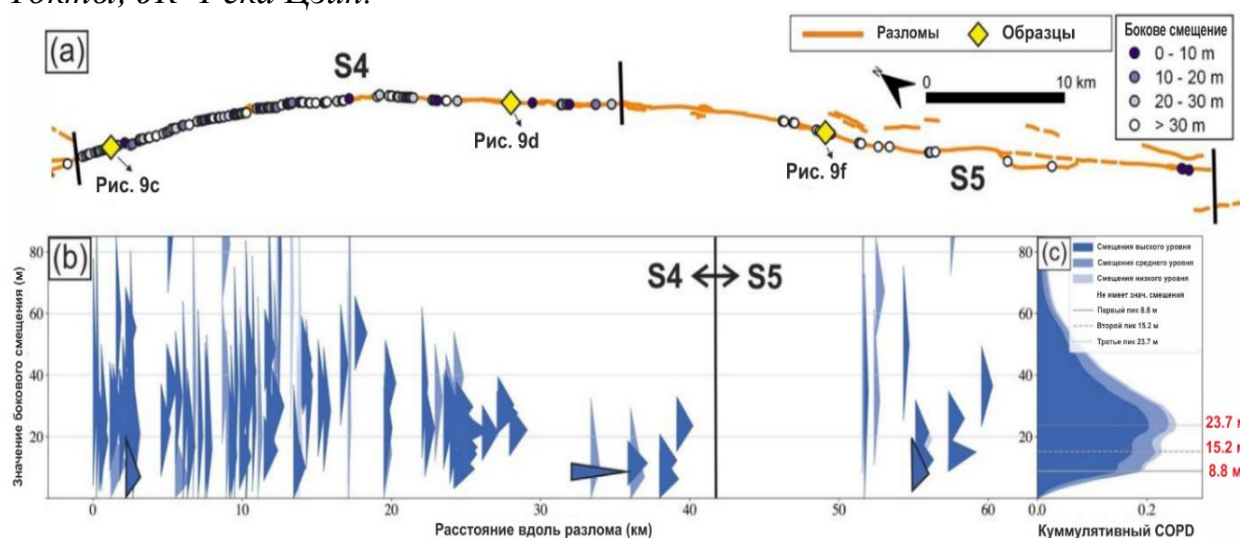
Рисунок 3.3. График плотности вероятности смещения (COPD) для участков S4 и S5 Джунгарского разлома (а). Кумулятивная плотность вероятности смещения (COPD) со значениями трех пиков отмечена цифрами красного цвета (с).
