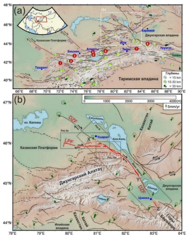
Рисунок 1.1. Топография, активные разломы, отдельные исторические землетрясения Тянь-Шаня и Джунгарии и векторы скорости GPS: (a) механизмы очагов землетрясений с M_w > 5 ; пронумерованные красные кружки - эпицентры разрушительных землетрясений: 1) Чаткальское 1946 г., 2) Суусамырское 1992 г., 3) Беловодское 1885 г., 4) Верненское 1887 г., 5) Чон-Кеминское 1911 г., 6) Чиликское 1889 г., 7) Нилки 1812 г. 8) Манасское 1906 г.; (b) красные линии - исследованные разрывные нарушения поверхности. Точки X и Y являются границами для трех основных участков (Северо-западный, центральный и юго-восточный). Охват спутниковых снимков Pléiades , используемых в нашем исследовании, простирается от точки X до Z. Голубые - города; KTF- Каратауский разлом, DNF-Жалайыр-Найманский разлом, AKF- Актасский разлом, DZF - Джунгарский разлом, TFF: Таласо-Ферганский разлом.
