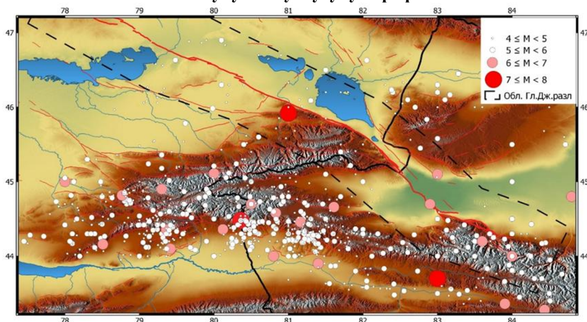
2.3-Сүрөт. Жунгариянын M_w \geq 4 болгон жер титирөөлөрүнүн эпицентрлеринин картасы (ЕМСА каталогу) жана активдүү жаракалары.
