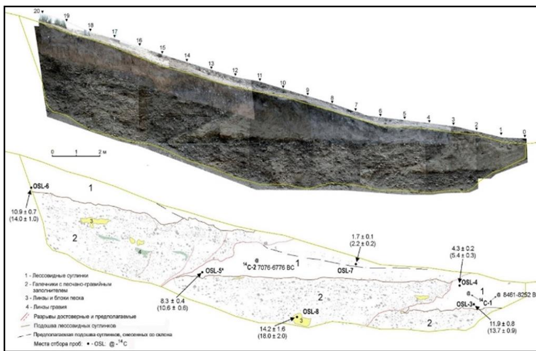
Рис. 3.1.1.6 - Общий вид траншеи, пройденной через уступ Центрально-Нарынского разлома.
