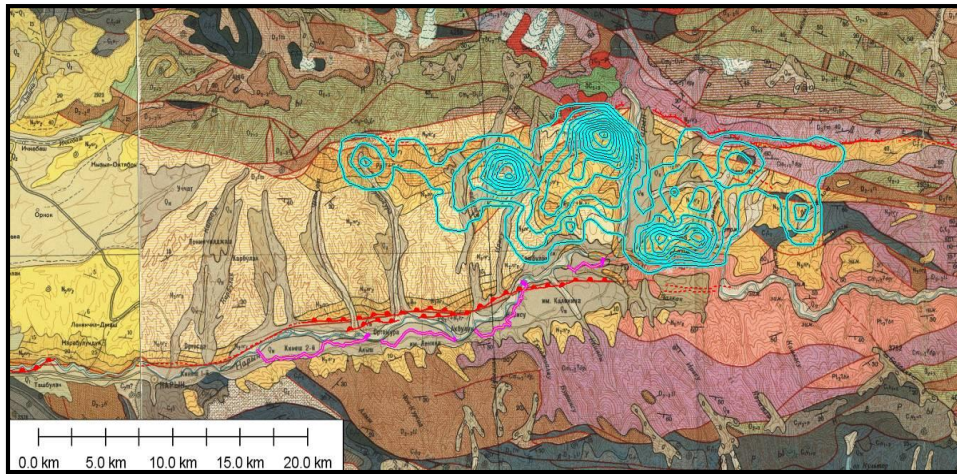
Рис. 4.1.3 - Сопоставление оползневой пораженности территории к северу от Центрально-Нарынского разлома с ее геологическим строением. Геология приведена по картам 1:200 000 [44].
