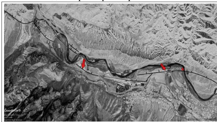
Рис. 3.20 - Активные разломы в пределах стройплощадки Университета. Красные стрелки - положение траншей. Цифры – номера траншей. Красная звездочка – места отбора образцов в уступе первой террасы р. Нарын.
