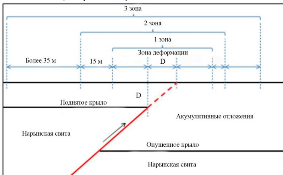
Рис. 4.4.2 - Зона влияния Центрально-Нарынского разлома в пределах территории Университета Ага-Хана по данным компании ARUP (Лондон, Англия - Фонды Института сейсмологии НАН КР).
