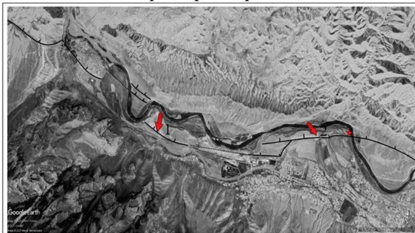
Рис. 3.20 - Активные разломы в пределах стройплощадки Университета. Красные стрелки - положение траншей. Цифры – номера траншей. Красная звездочка – места отбора образцов в уступе первой террасы р. Нарын.
