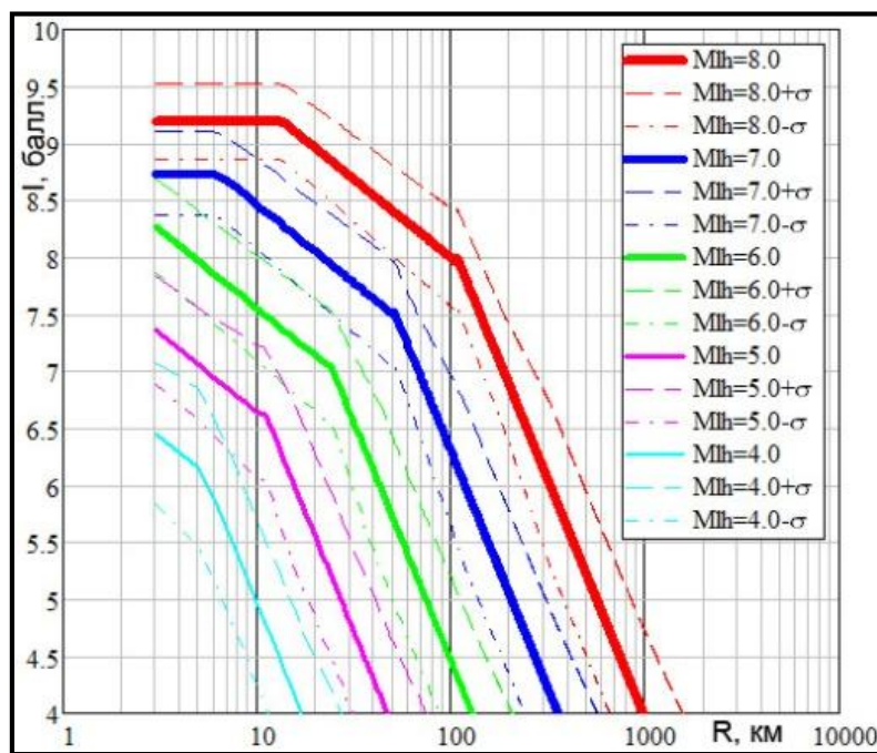
Рис. 4.2.1 - Зависимость сейсмической интенсивности от расстояния до источника с магнитудой M_{LH} для землетрясений со взбросовой кинематикой подвижки в очаге землетрясения. Графики построены С.А. Перетокиным (НП ЭЦ РОПР) по данным Ф.Ф. Аптикаева (ИФЗ РАН) [12].
