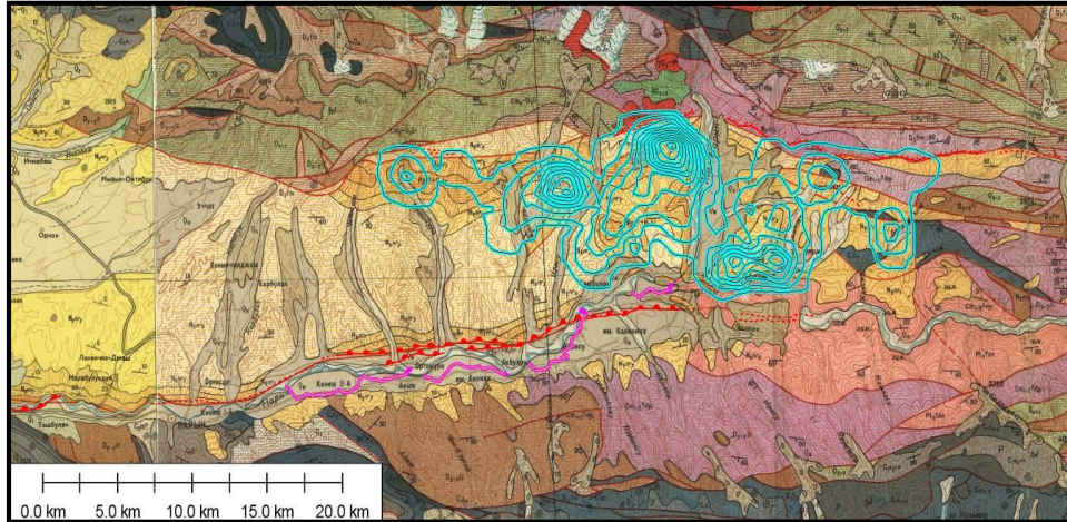
Рис. 4.1.3 - Сопоставление оползневой пораженности территории к северу от Центрально-Нарынского разлома с ее геологическим строением. Геологическое строение района приведена по картам 1:200 000 [44].
