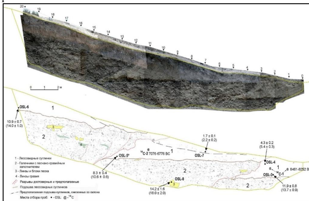
Рис. 3.1.1.6 - Общий вид траншеи, пройденной через уступ Центрально-Нарынского разлома.
