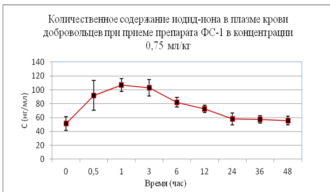
Рис. 3.16. Усредненный фармакокинетический профиль иодида-иона в плазме крови добровольцев после однократного орального приема
