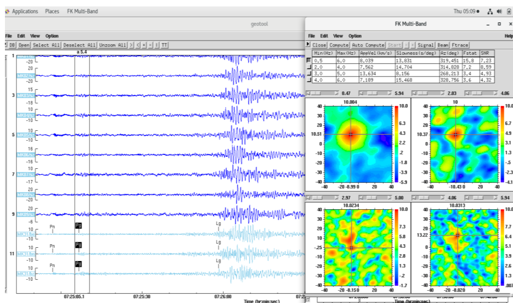
Рисунок 1.6 - Пример записи (слева) и нахождения азимута прихода и кажущейся скорости (справа) сейсмических сигналов по группе Маканчи.
