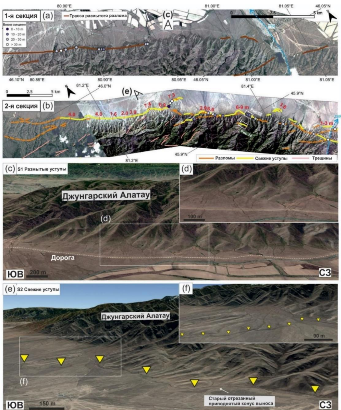
Рисунок 3.4 – Изображения спутника Pléiades, показывающие (а) сегмент 1 и (б) сегмент 2 Джунгарского разлома с нанесенными на карту трассами разломов и смещениями (местоположения см. на рисунке 3.3, TTR: р. Тентек, ZMR: р. Жаманты). Высоты свежих уступов отмечены красным текстом с короткими красными линиями, показывающими измеренные местоположения. (с) и (е) — спутниковые снимки Google Earth, направленные под углом к юго-западу вдоль участков 1 и 2, с крупным планом, показанным на (d) и (f) соответственно, показывая разный уровень деградации уступа и морфологию на фронте хребта. между этими двумя разделами.
