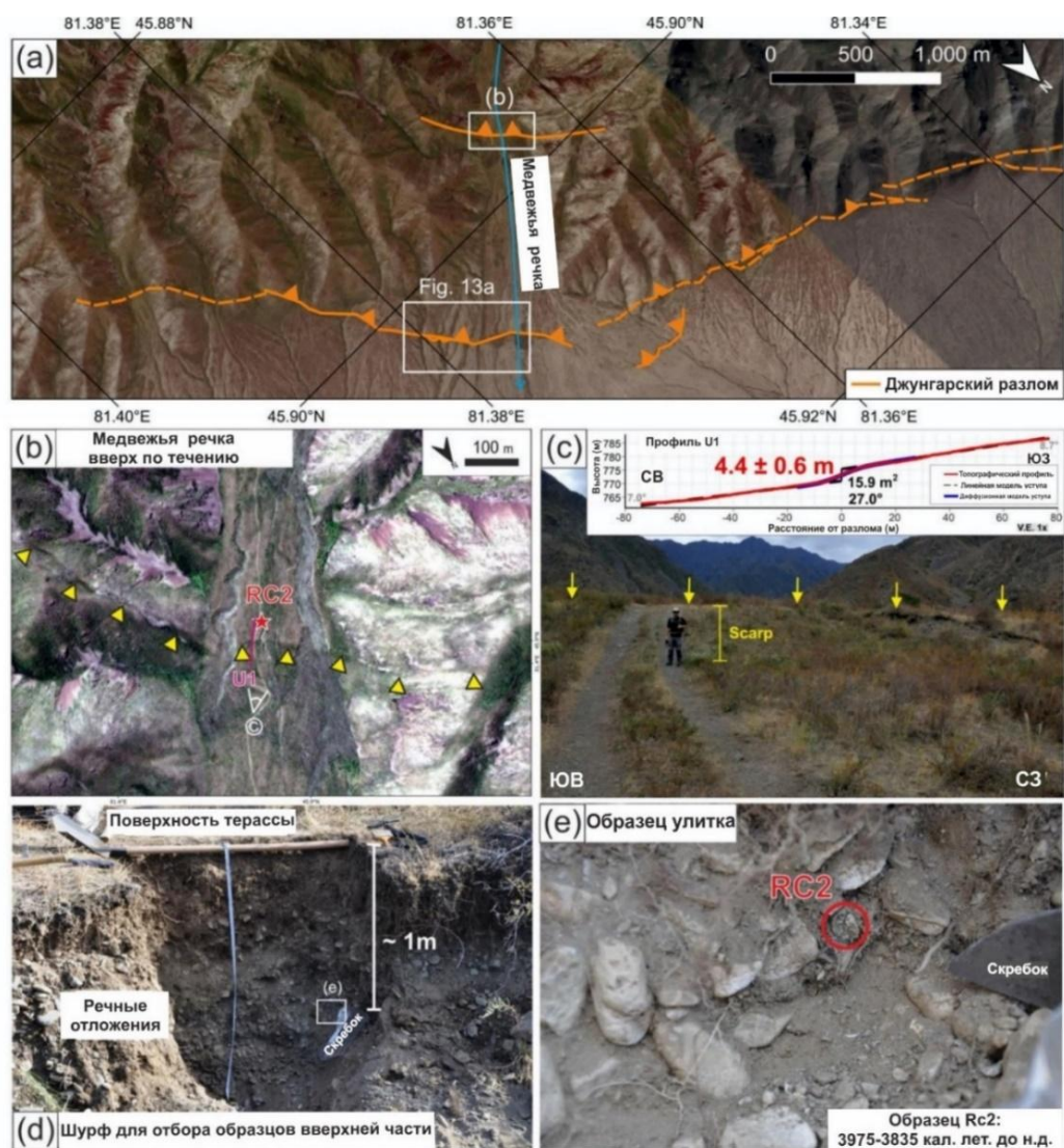
Рисунок 3.11 - (a) Ортотрансформированные изображения Pléiades, показывающие второй уступ (желтые стрелки) вверх по течению от участка Медвежья река (81.36° В.Д., 45.90° С.Ш.). Место отбора образца RC2 отмечено красной звездой, короткая красная линия - профиля dGPS. (c) Полевая фотография уступа с топографическим профилем dGPS и результатами морфологического датирования уступа, показанными на вставке. (d, e) Полевые
