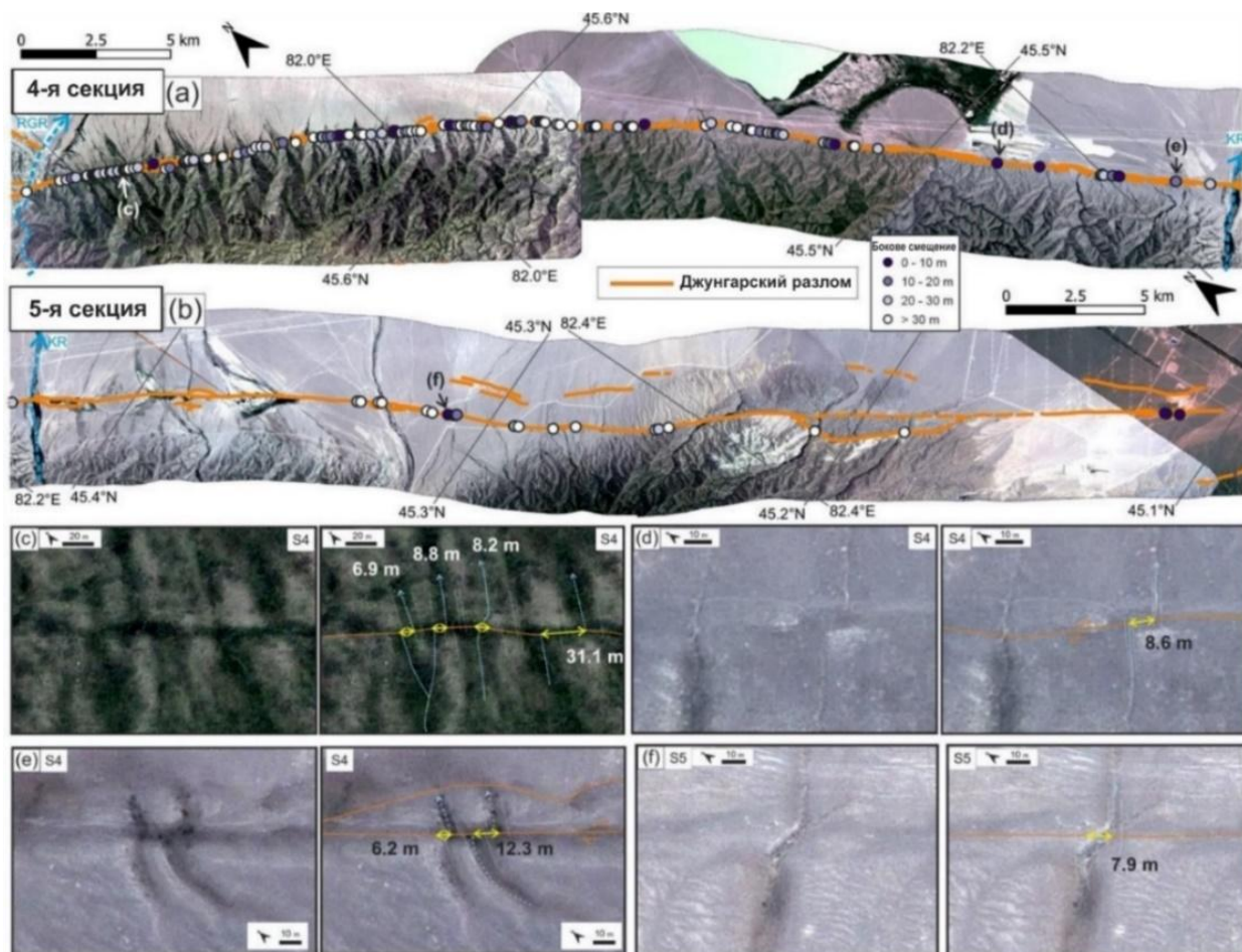
Рисунок 3.6 - Ортотрансформированные снимки Pléiades, показывающие секций S4(a) и S5(b) Джунгарского разлома с нанесенными на карту трассами разломов и местами измерения смещения. (c–f) Снимки Pléiades крупным планом, показывающие мельчайшие высококачественные смещенные русла вдоль участков S4 и S5 со смещениями в метрах. В примере (e) показаны смещенные близко расположенные русла, вероятно единичные события и кумулятивные смещения. В точке (e) имеется второй разлом, так что измеренное смещение может недооценивать смещение при землетрясении, и такого рода измерения будут исключены из графика плотности вероятности и анализа кумулятивной плотности вероятности смещения (COPD).
