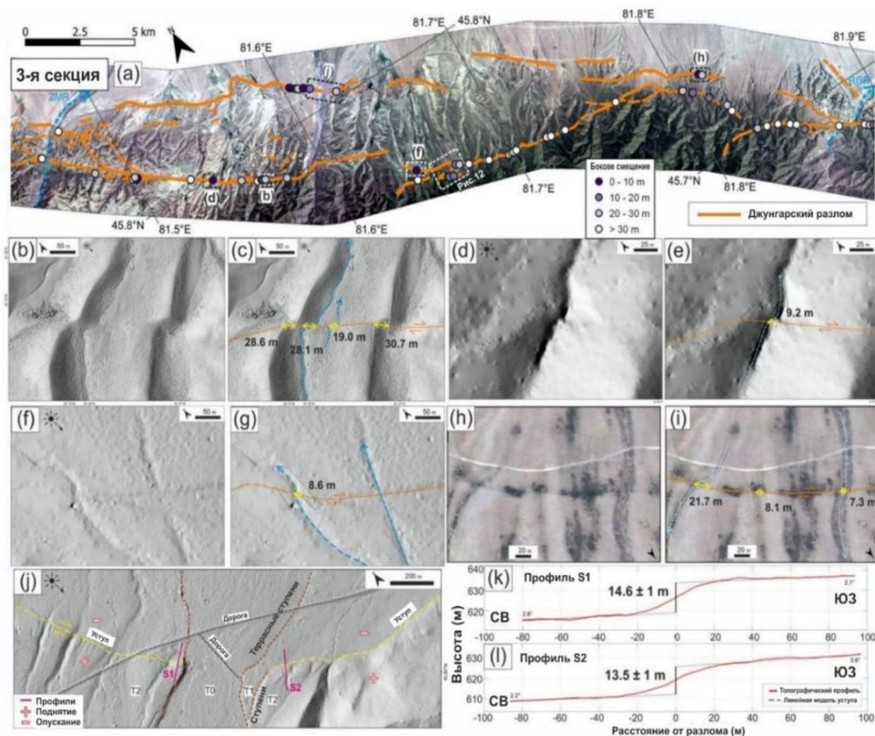
Рисунок 3.8 - (а) Ортотрансформированное изображение Pléiades, показывающий участок S3 Джунгарского разлома (см. местоположение на рисунок 3.3) с нанесенными на карту трассами разломов и измерениями смещения. (b)-(i) Ортотрансформированная и затененная топография, полученная из изображений Pléiades боковых смещенных русел на S3 с аннотированными величинами смещения, см. «а» для местоположений. (j) Топография с затененным рельефом, полученная из изображений Pléiades, показывающая террасы T2-T0, от старых к молодым, и уступы длиной ~ 14 м вдоль северной ветви разлома с отмеченными местоположениями двух профилей (S1 и S2). (k, l) Топографические профили S1 и S2 из ЦМР, полученных с помощью Pléiades, с указанием высот.
