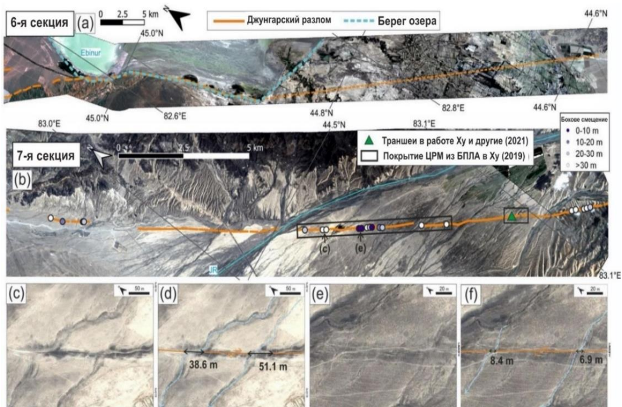
Рисунок 3.5 - Ортотрансформированное изображение Pliades участков 6 (a) и 7 (b) с нанесенными на карту трассами разломов и местами измерения смещений. Максимальная протяженность береговой линии Эбинура показана синей пунктирной линией (a). Расположение траншеи и покрытие снимков с дронов высокого разрешения отмечены буквой (b) [35].
