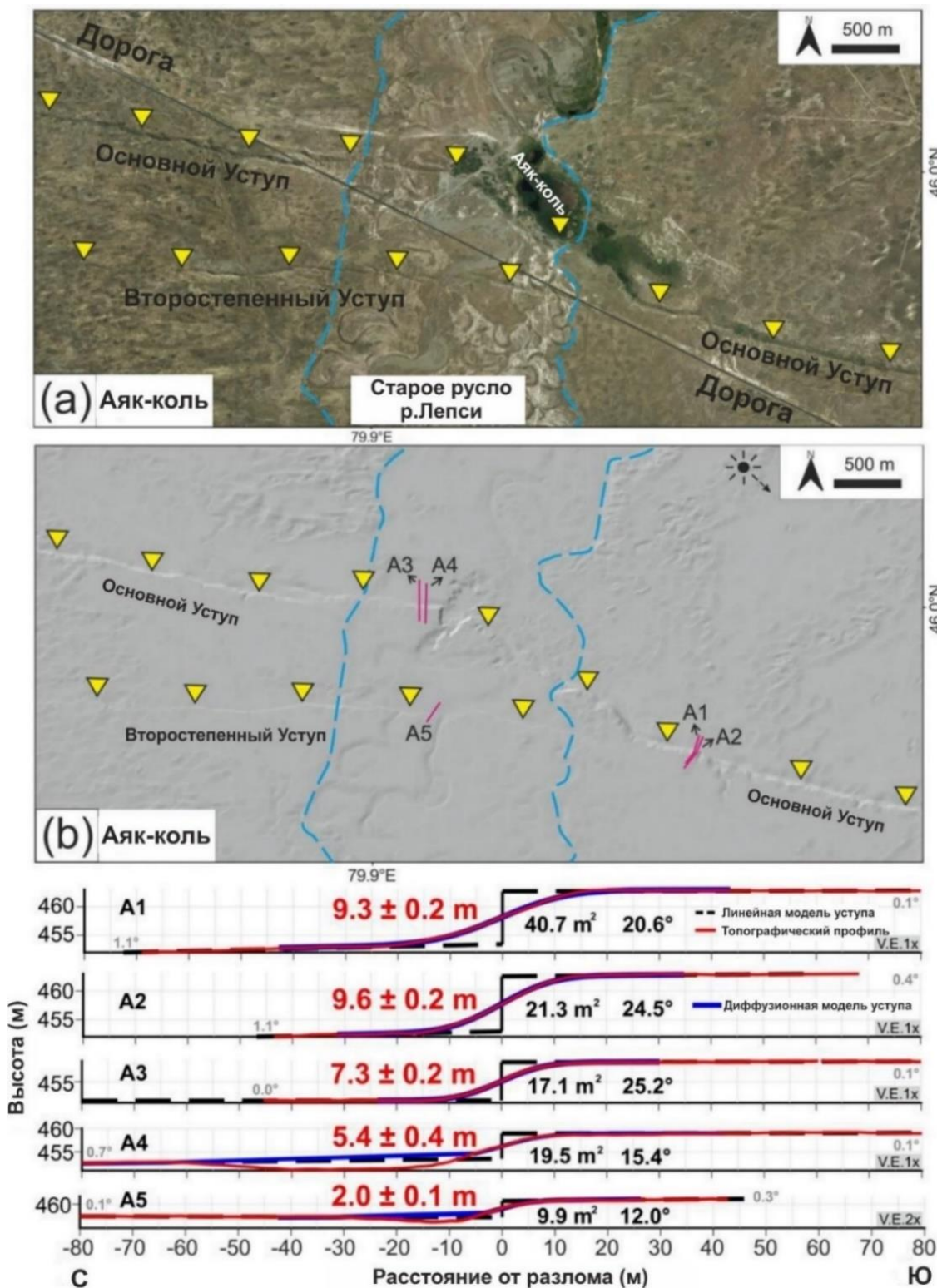
Рисунок 3.2 – Лепсинский разлом в районе оз. Аякколь: (а) спутниковый снимок Bing Map, (б) рельеф ЦМР НМА; синие пунктирные линии - старое русло р. Лепси; желтые стрелки - свежие уступы [24]. Ниже показаны пять
