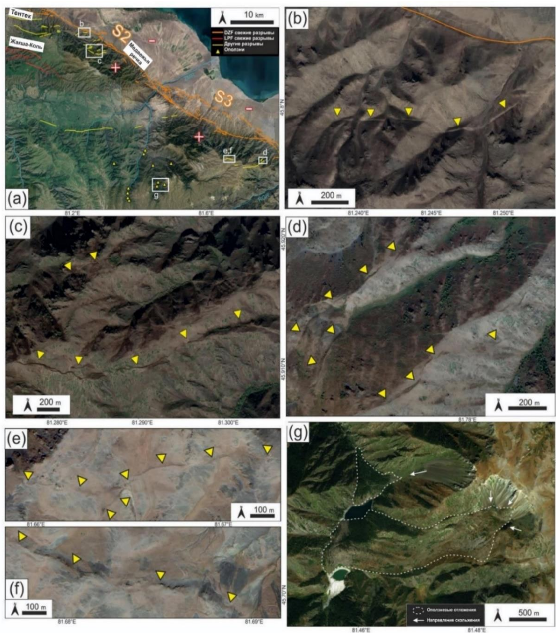
Рисунок 3.13 - (a) Снимок BingMap, показывающий северный Джунгарский Алатау с нанесенными на карту следами разломов и оползней. (b-
