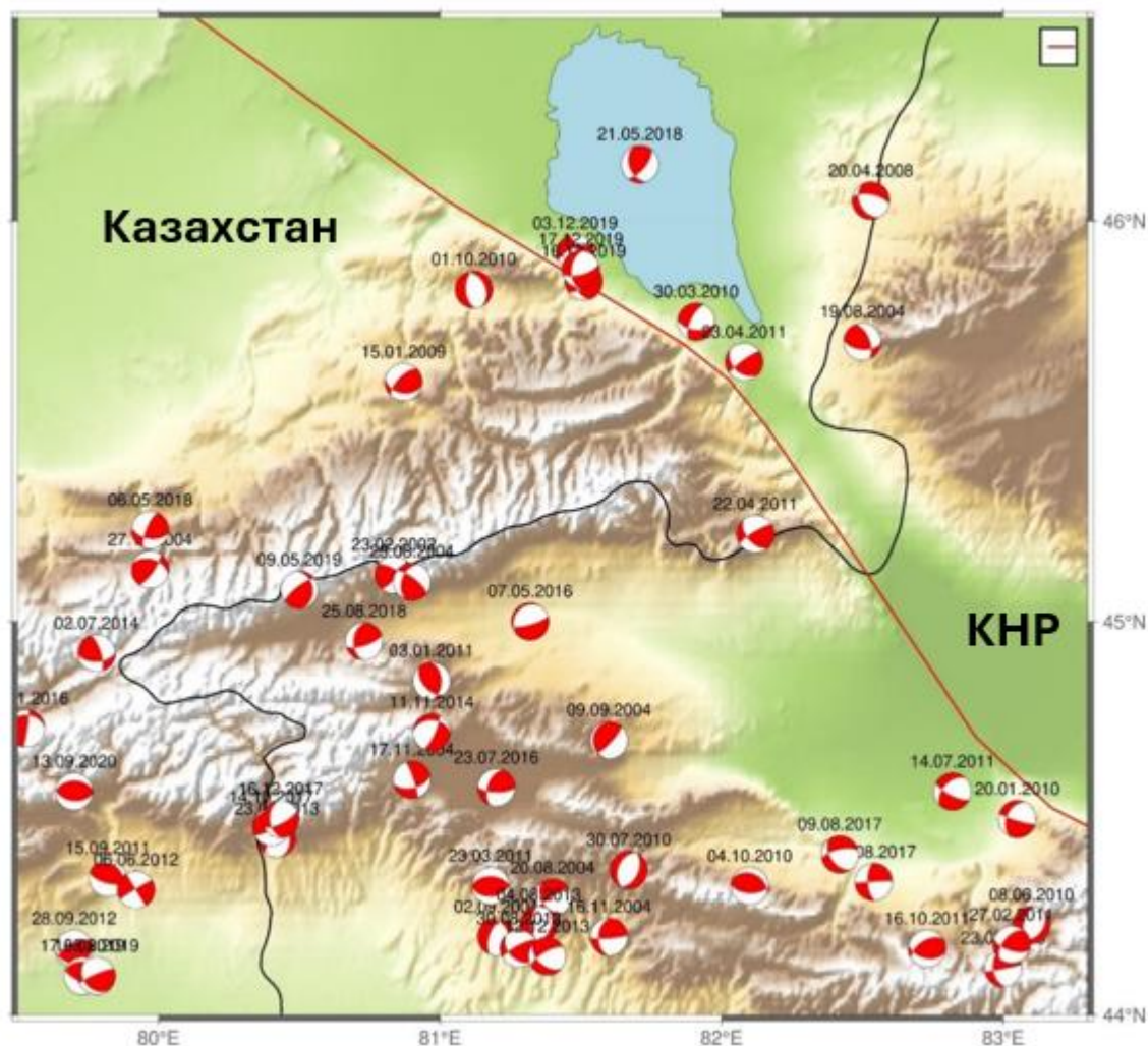
Рисунок 2.13 – Карта механизмов очагов землетрясений Джунгарии по данным каталога ННЦСНИ МЧС РК и ИГИ НЯЦ РК (красная линия – главный Джунгарский разлом).
