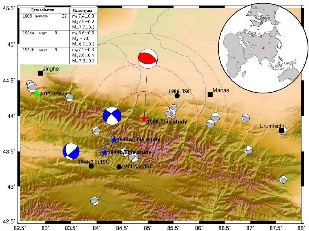
Рисунок 4.4 - Фокальные механизмы и результаты перелокализации Манасского (1906 г., красный цвет) и Синьянских землетрясений (1944г., синий цвет) [102].
