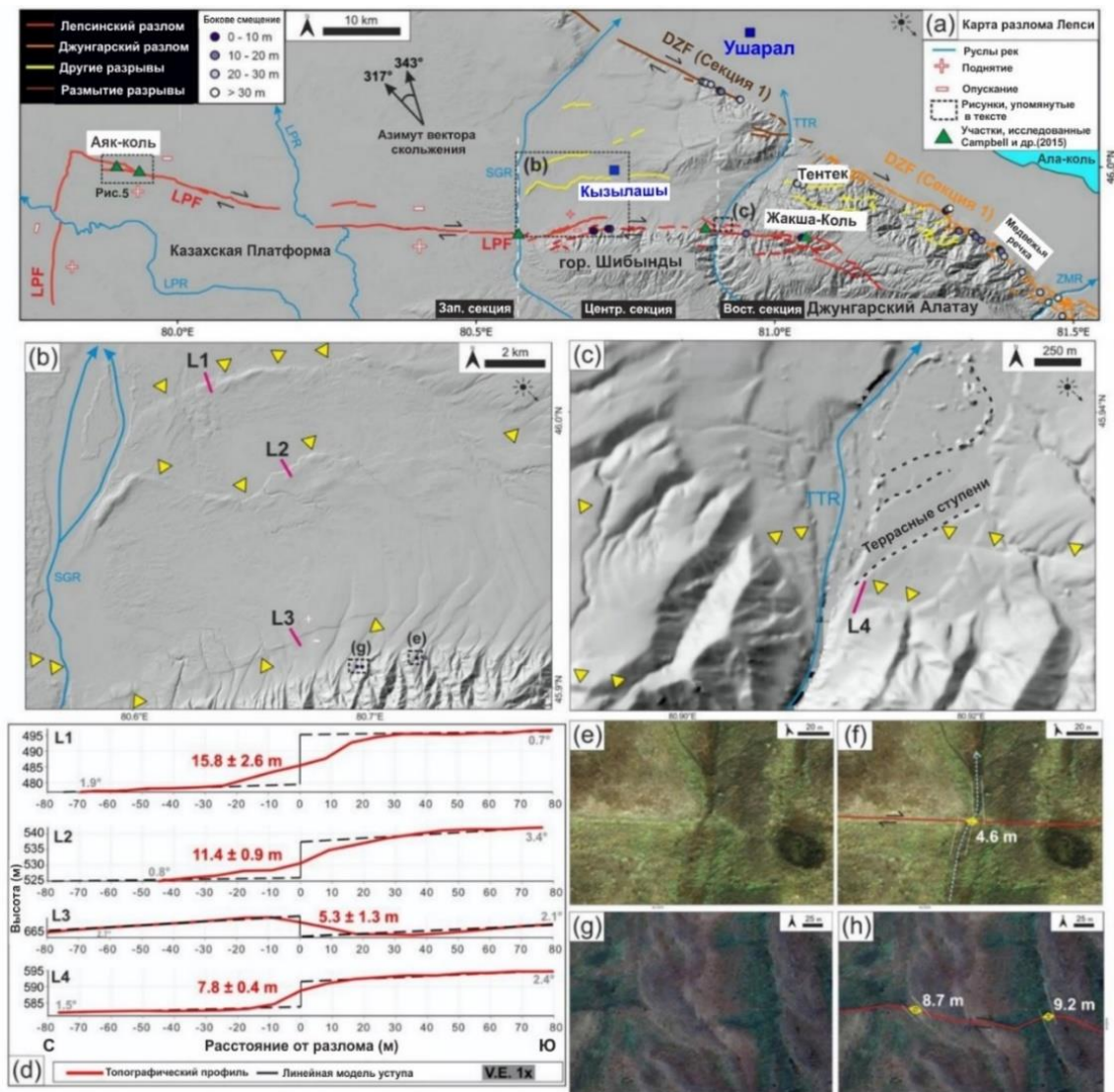
Рисунок 3.1 – Карта района Лепсинского и Джунгарского разлома.
