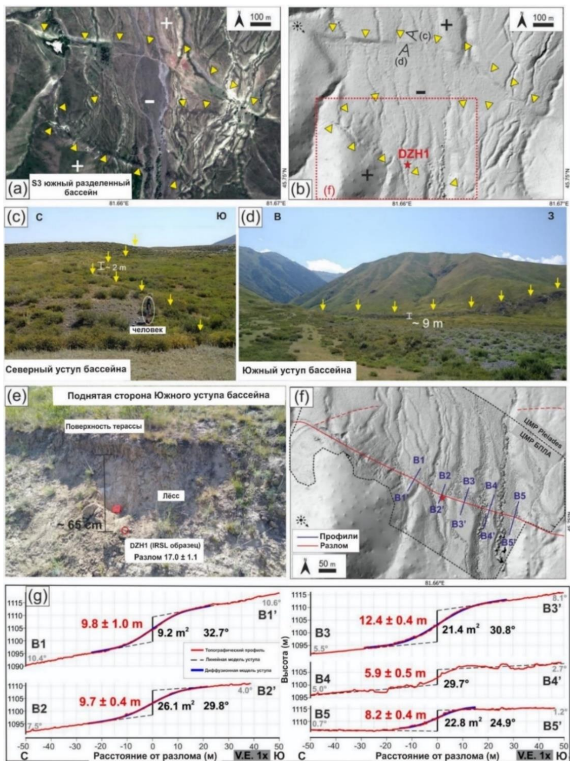
Рисунок 3.9 - Впадина вдоль Джунгарского разлома на сегменте S3 (местоположение см. на рисунке 3.8а). (а) Ортотрансформированные изображения Pléiades с уступами, показанными желтым цветом. (б) Топография с затененным рельефом, полученная из снимков Pléiades, с обозначением места отбора образца DZH1 (красная звездочка). (с и d) Полевые фотографии
