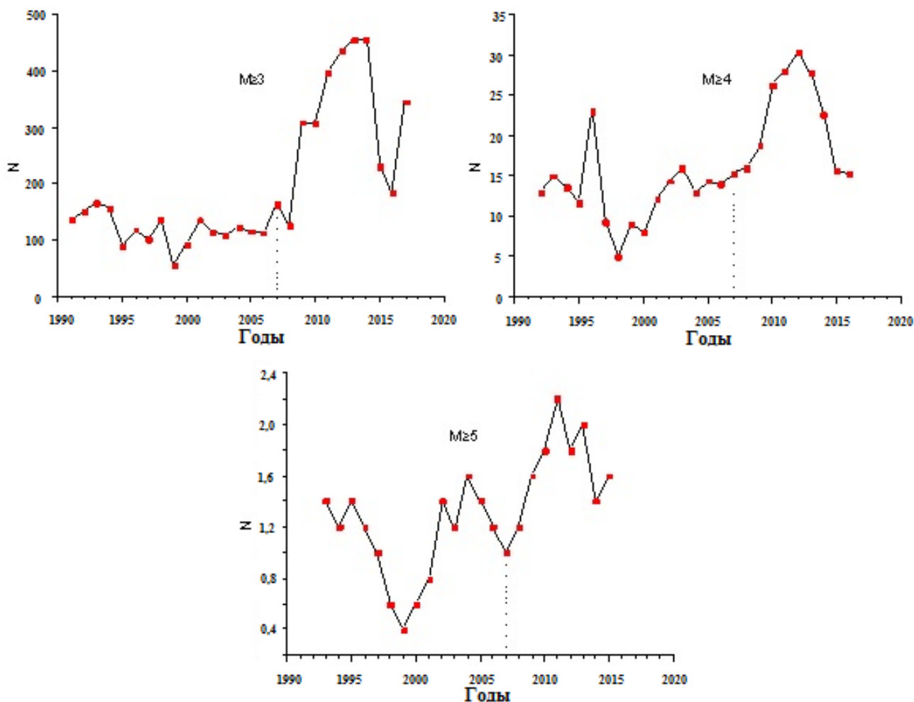
Рисунок 4.7 - Графики годовых вариаций землетрясений в разных магнитудных диапазонах [193].
