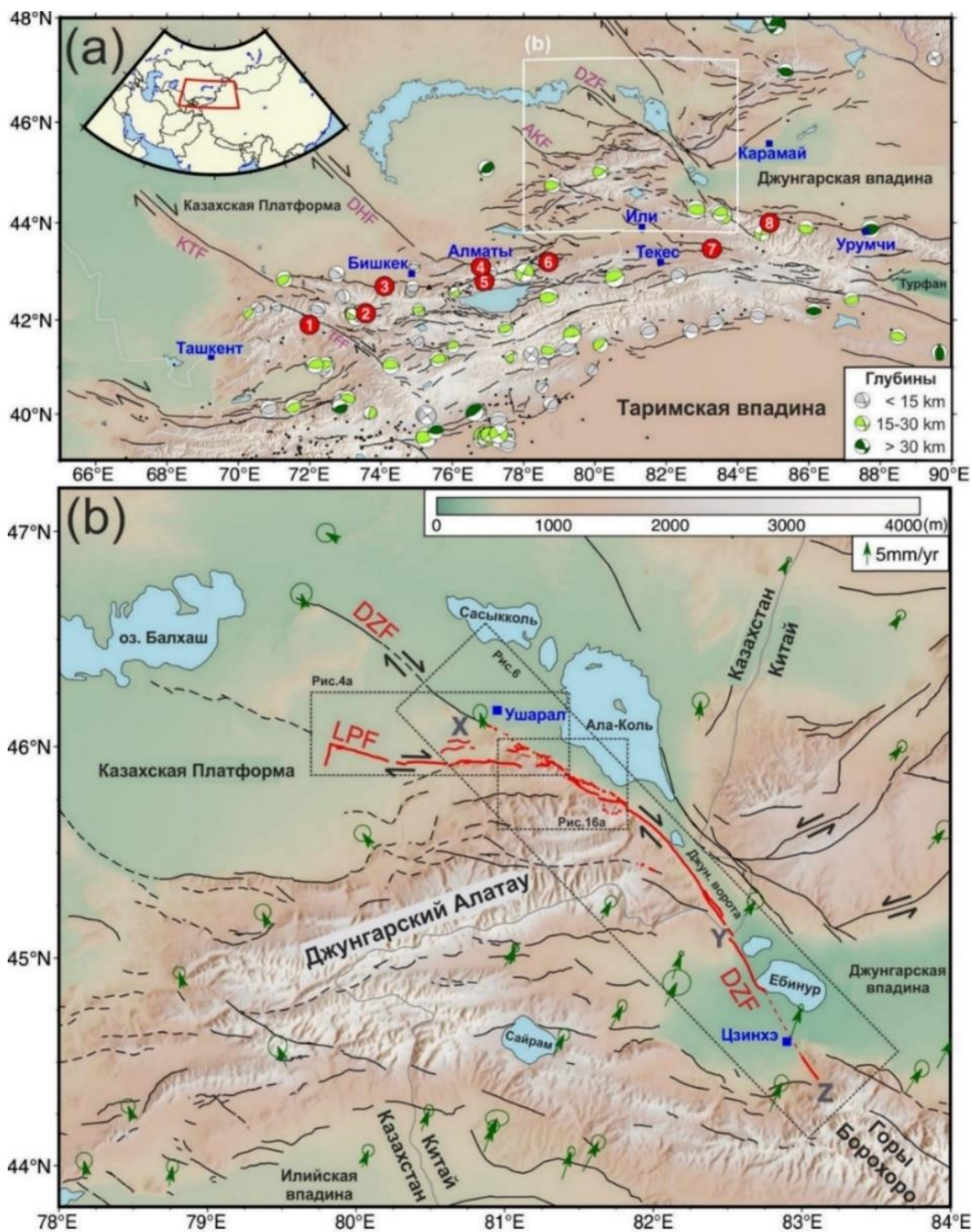
Рисунок 1.1 - Топография, активные разломы и отдельные исторические землетрясения Тянь-Шаня и Джунгарии и векторы скорости GPS [60, 74].
