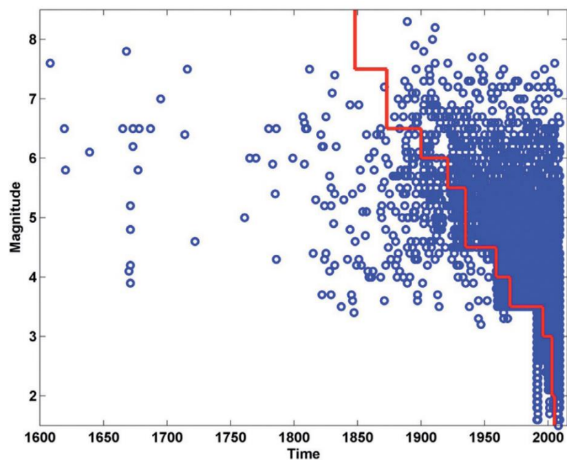
Рисунок 2.1 - Анализ полноты (красная линия) каталога ЕМСА по магнитуде MLH [153].
