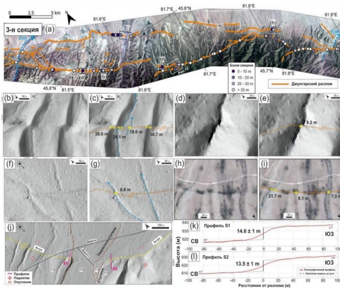
Рисунок 3.8 - (а) Ортоотраформированное изображение Pléiades, показывающий участок S3 Джунгарского разлома (см. местоположение на рисунок 3.3) с нанесенными на карту трассами разломов и измерениями смещения. (b)-(i) Ортоотраформированная и затененная топография, полученная из изображений Pléiades боковых смещенных каналов на S3 с аннотированными величинами смещения, см. «а» для местоположений. (j) Топография с затененным рельефом, полученная из изображений Pléiades, показывающая террасы T2-T0, от старых к молодым, и уступы длиной ~ 14 м вдоль северной ветви разлома с отмеченными местоположениями двух профилей (S1 и S2). (k, l) Топографические профили S1 и S2 из ЦМР, полученных с помощью Pléiades, с указанием высот.
