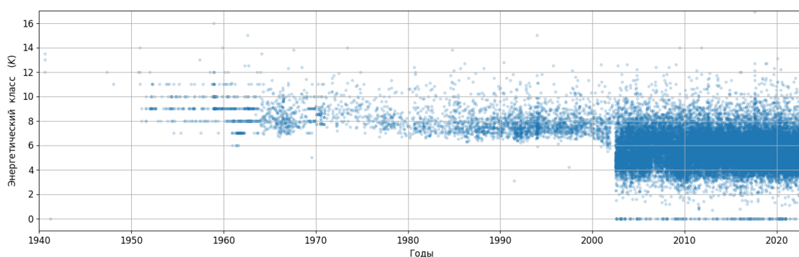
Рисунок 2.4 – График полноты каталога землетрясений территории Джунгарии.
