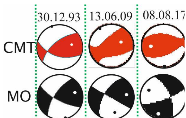
Рисунок 4.6 - Сопоставление решений механизма очага и СМТ для Текелийских землетрясений и Борохорского землетрясения
