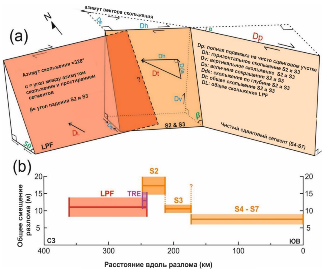
Рисунок 4.1 - (а) Эскиз, показывающий упрощенную геометрию разлома, включая Лепсинский разлом и сегменты S2-S7 Джунгарского разлома. Подвижки на участках S2 и S3, которые включают существенные вертикальные и горизонтальные составляющие, оцениваются с учетом постоянного азимута вектора подвижки 328^\circ для всех участков; (б) смещения на сегментах S2-S7 Джунгарского разлома (оранжевый) и Лепсинского (красный) и на разломе восточнее р. Тентек (TRE).
