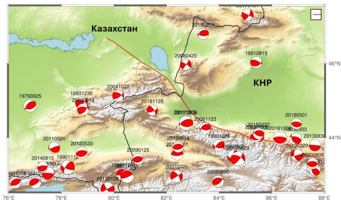
Рисунок 2.12 – Карта механизмов очагов землетрясений Джунгаро-Северо-Тянь-Шанского региона по данным GСMT [101]. (красная линия – главный Джунгарский разлом).
