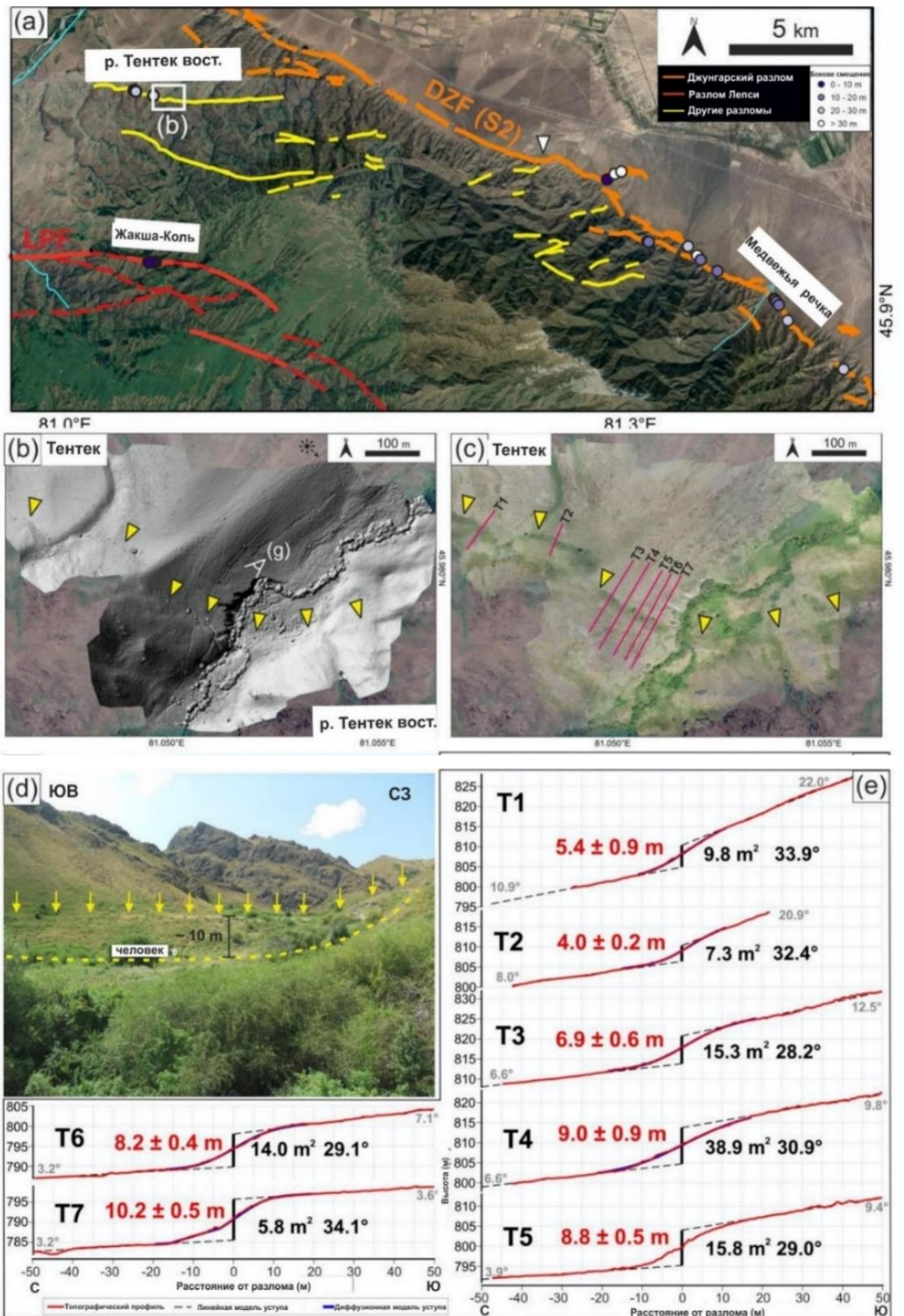
Рисунок 3.12 - (а) Снимок Bing Map, показывающий зону перехода между Лепсинским и Джунгарским разломами. Белым треугольником отмечен переход,
