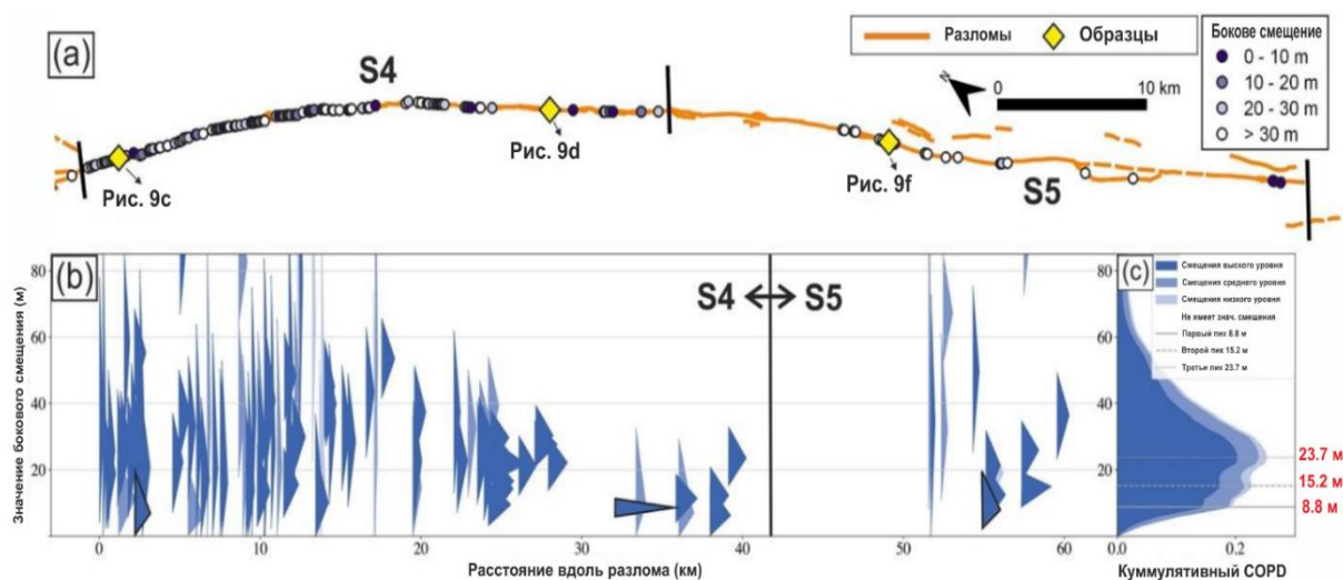
Рисунок 3.7 - Трасса участков S4 и S5 Джунгарского разлома (сверху) и график плотности вероятности смещения (COPD снизу) для 113 правосторонних каналов вдоль участков S4 и S5.
