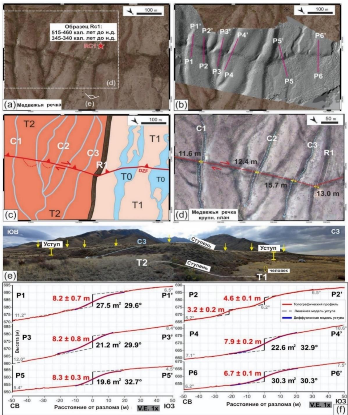
Рисунок 3.10 - (а) Ортотрансформированные снимки Pleiades, показывающие уступы и смещенные русла разлома на участке Медвежья река (81.37° в.д., 45.90° с.ш.) в пределах участка S2 (см. рисунок 3.11). Местоположение образца RC1 (красная звезда) и его возраст указано на рисунке (а). ЦМР, полученный с помощью БПЛА, показывающая тот же вид, что и на рисунке (а) и местоположения топографических профилей показаны на рисунке (b). Рисунок (c) - геоморфологическая карта, показывающая протяженность
