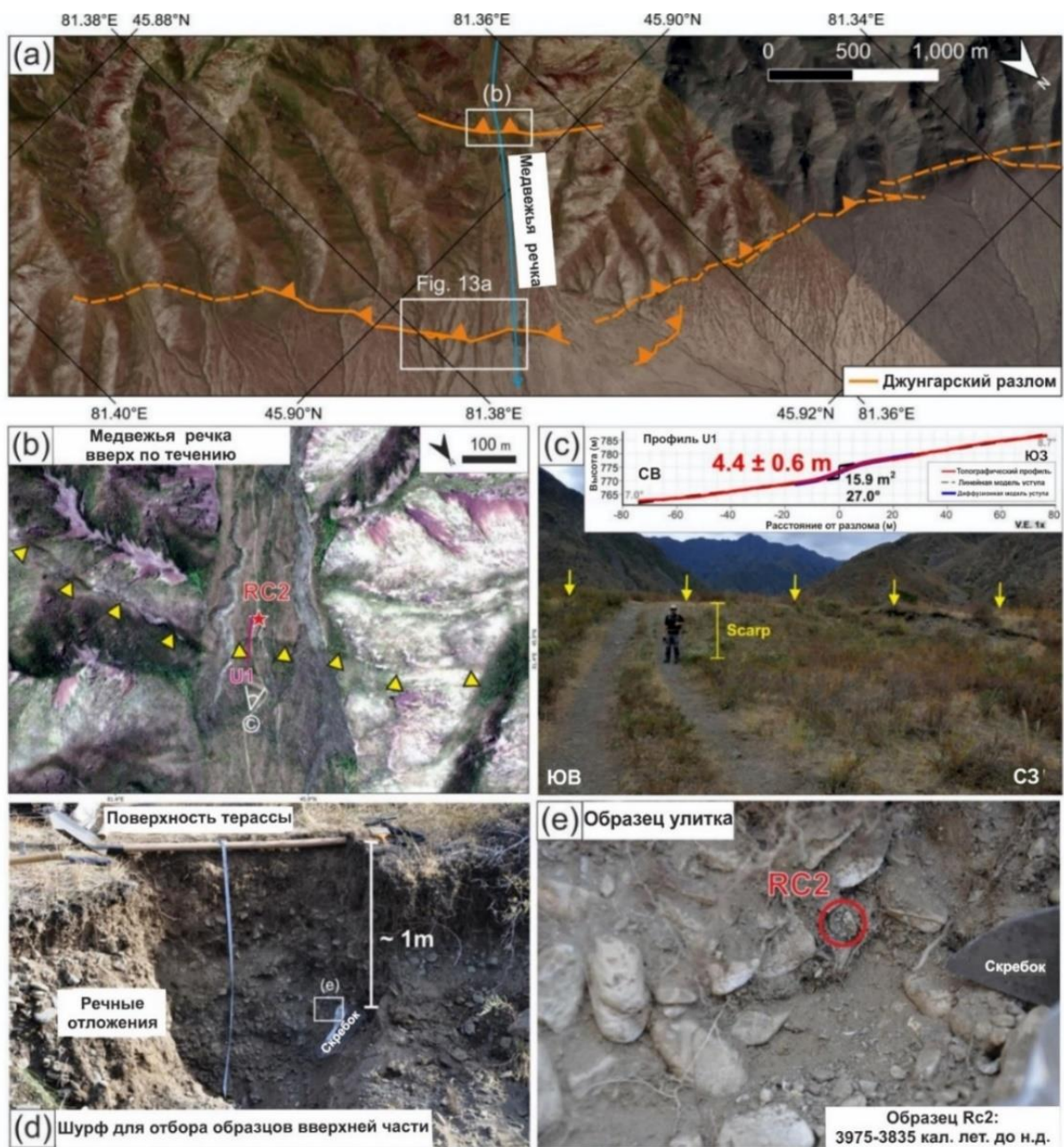
Рисунок 3.11 - (а) Ортотрансформированные изображения Pléiades, показывающие второй уступ (желтые стрелки) вверх по течению от участка Медвежья река ( 81.36^\circ в.д., 45.90^\circ с.ш.). Место отбора образца RC2 отмечено красной звездой, короткая красная линия - профиля dGPS. (с) Полевая фотография уступа с топографическим профилем dGPS и результатами морфологического датирования уступа, показанными на вставке. (d, e) Полевые фотографии шурфа и образца брюхоногих моллюсков RC2 (красный кружок) с указанием калиброванным радиоуглеродным возрастом.
