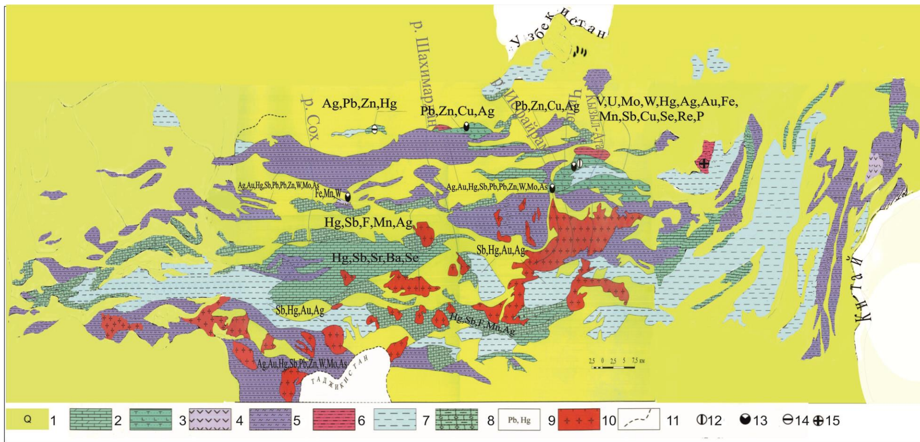
Рис. 1. Схематическая карта рудоносных стратифицированных формаций Туркестано-Алая
