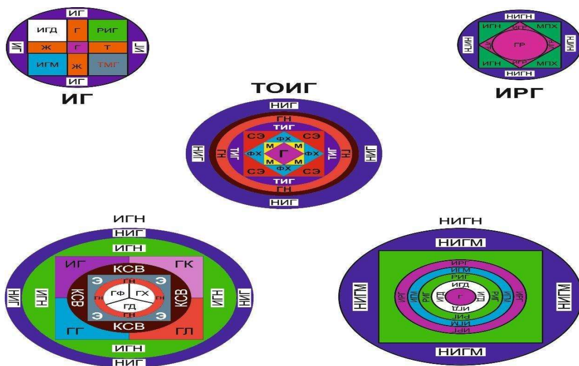
Рисунок 3. Обоснование круговыми диаграммами этапов становления нового научного направления НИГ на примере месторождений полезных ископаемых во взаимосвязи с грунтоведением, инженерной и экологической геологией (ИГ), инженерно-рудничной геологией, технической мелиорацией грунтов, геологической, физико-химической, механико-математической, социально-экономической и основами теории инженерной геологии (ТОИГ), гидрогеологии, геокриологии, геогидрологии, геоэкологии, геонимии, катастрофоведения, инженерной геонимии (ИГН), которые позволяют создать основы Общей и Единой теории Земли
