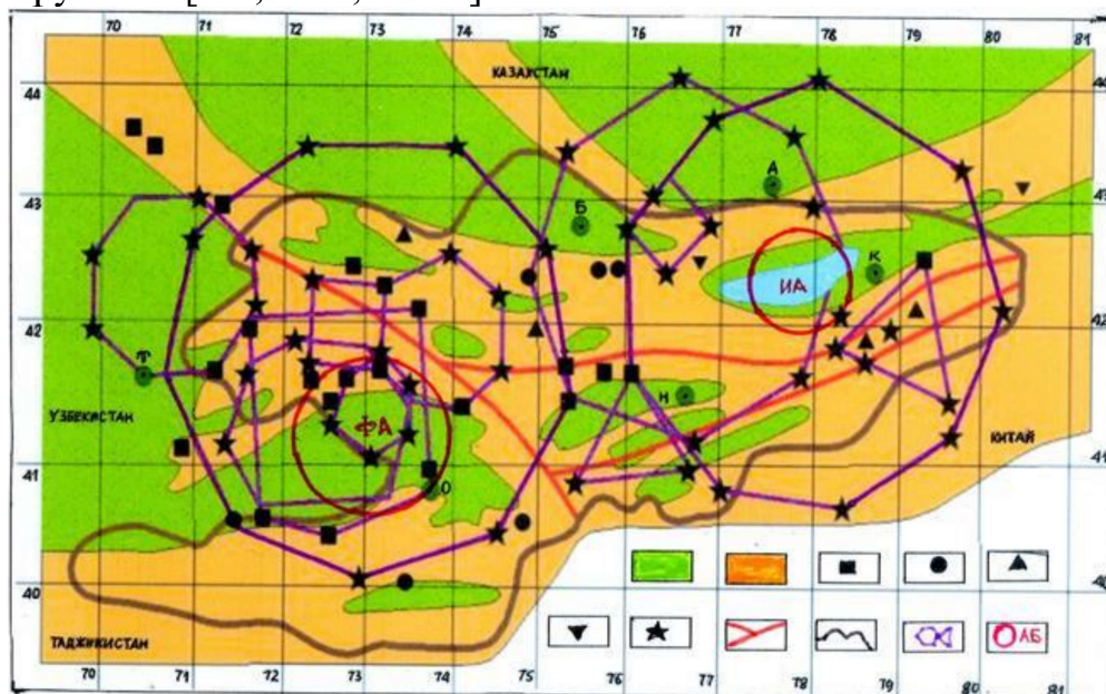
Рисунок 23. НИГ карта полигоногранной типизации и прогнозирования новых точечных узлов вероятной концентрации месторождений рудных ископаемых
