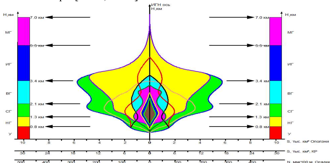
Рисунок 25. НИГ модель вертикальной повысотной закономерности распространения, типизации и прогноза георисков от оползней, атмосферных осадков, активизирующихся при освоении полезных ископаемых на территории Кыргызстана.
