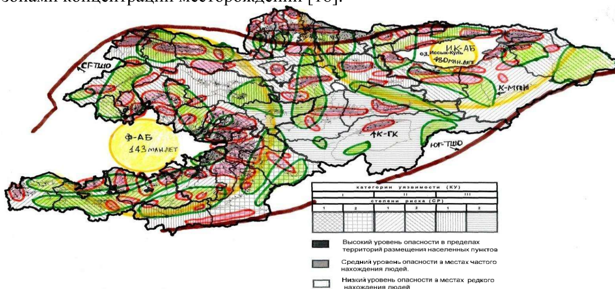
Рисунок 18. НИГ карта-схема типизации концентрации георисков (красные контуры) и месторождений полезных ископаемых (зеленые ареалы) на карте по-районного прогнозирования категорий уязвимости (КУ), степени риска (СР) и уровня опасности (УО) от возможной активизации многоступенчатых катастроф: коричневые толстые линии, границы (СГ-ТШО) северного и южного (ЮГ-ТШО) Тянь-Шаньского эпиплатформенного орогена; круги закрашенные в желтый цвет мегаструктуры центрального типа представленные мегаструктурами центрального типа от ударных столкновений 480 млн. лет тому назад с Иссык-Кульским и, 142 млн. лет. тому назад с Ферганскими астероидоблемами с планетосферами Кыргызстана.
