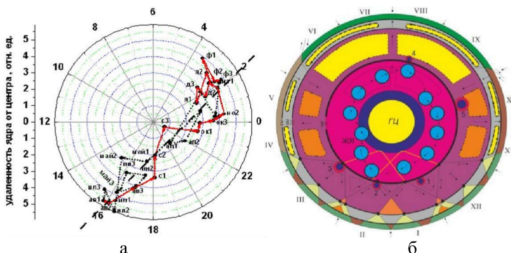
Рисунок. 7. НИГ инструментальная (а) и инновационная (б) модель орбитального круглогодичного импульсного вращения твердого ядра внутри жидкой планетосферы вокруг геометрического центра Земли, трансформирующего копоненты полигрунтов в геосферах и активизирующие геориски гравиинертного, сейсмотектонического и электромагнитного характера и участвующие в формировании, миграции и концентрации полезных ископаемых на Геоиде и его субчастях
