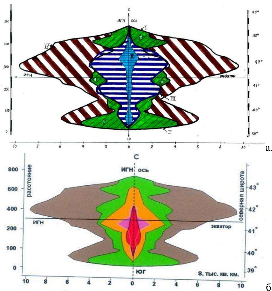
Рисунок 24. НИГ латеральная поширотная модель закономерности распространения, типизации и прогноза георисков, воздействующих при освоении полезных ископаемых на рудники, населенные пункты Кыргызстана, геономы: а) 1-долинности, 2-олененности, 3-мерзлотности, 4-орогенности; б) коричневый орогенности, зеленый-долинности, геориски от оползней светло-фиолетовая 1-ой, красная 2-ой, оранжевая 3-ей категории уязвимости
