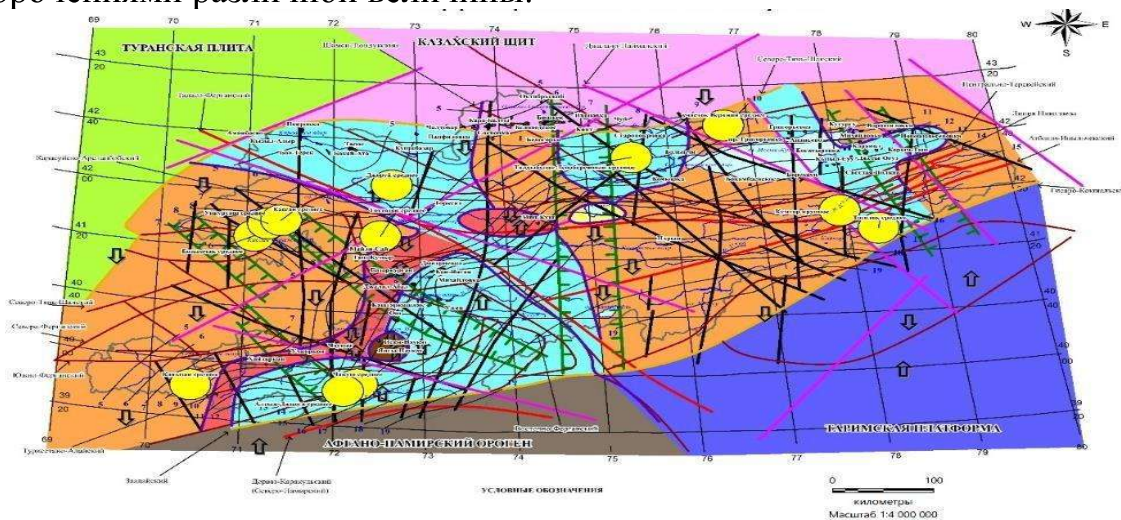
Рисунок. 10. НИГ карта закономерностей распространения, типизации и прогнозирования георисков, несущих угрозу рудникам и карьерам на примере месторождений золота на территории Кыргызского Тянь-Шаня и Памиро-Алая
