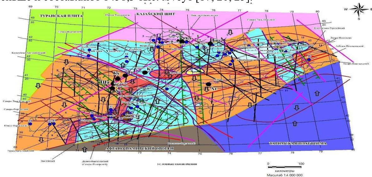
Рисунок. 8. НИГ карта закономерностей распространения, типизации и прогнозирования георисков, несущих угрозу при освоении и эксплуатации месторождений подземных вод (синие кружочки) и трансформируемые в поле палеопрочности полигрунтов активными границами поливергентных неотектонических движений и их структурами, разломами и линеаментами, разрушающими литосферу Кыргызского Тянь-Шаня и Памиро-Алая
