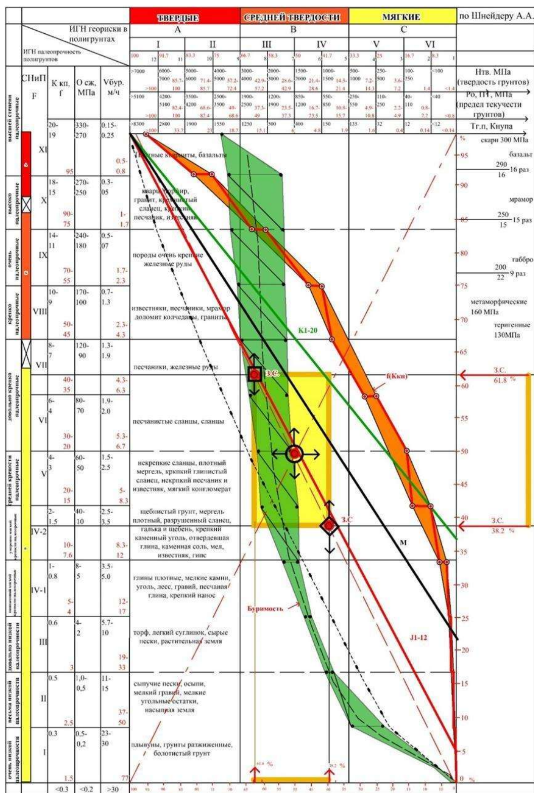
Рисунок 21. НИГ универсальная шкала закономерности изменчивости крепости и податливости полигрантов для оценки и прогнозирования трансформации георисками поля палеопрочности планетосфер их субчастей.
