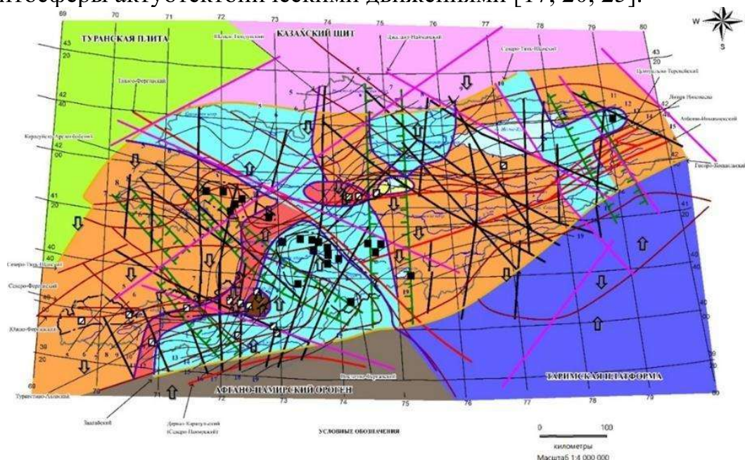
Рисунок 12. НИГ карта закономерностей распространения, типизации и прогнозирования георисков, несущих при освоении и разработке угрозу карьерам и шахтам на примере месторождений углей, нефти и газа на территории Кыргызского Тянь-Шаня и Памиро-Алая
