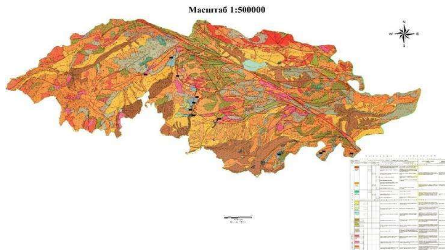
Рисунок. 13. НИГ карта закономерностей инженерно-геологических формационных условий распространения, типизации и прогнозирования георисков, воздействующих на карьеры и шахты на примере месторождений углей на территории Жалал-Абадской области Кыргызстана.
