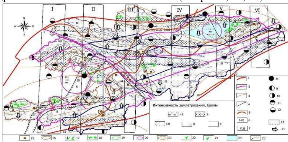
Рисунок 14. НИГ карта типизации георисков, несущих угрозу карьерам и шахтам при освоении угольных бассейнов с прогностическими эпицентрами районов ожидаемых землетрясений, направлениями и величинами вергентных неотектонических и современных движений в земной коре Кыргызского Тянь- Шаня и Памиро-Алая
