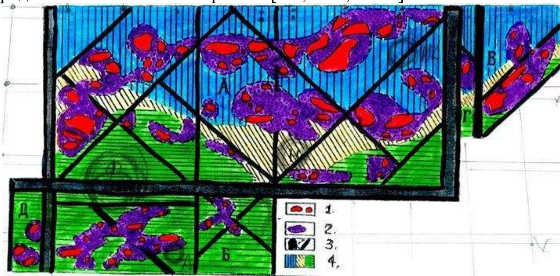
Рисунок 22. НИГ карта квазисимметрической линейно-нелинейной типизации известных проявлений рудной минерализации и выявления перспективных для поиска и разведки новых площадей оруденения на территории Кыргызского Тянь-Шаня и Памиро-Алая
