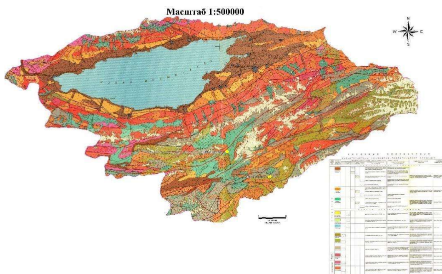
Рисунок 11. НИГ карта закономерностей инженерно-геологических формационных условий распространения, типизации и прогнозирования георисков, воздействующих на карьеры и шахты на примере месторождений золота на территории Ыссык-Кульской области Кыргызстана
