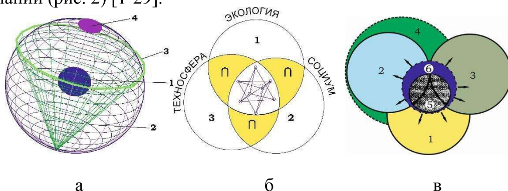
Рисунок 2. Обоснование на базе моделей ноосферы Вернадского В.И. (1935) и Трофимова В.Т., Королева В.А. (2014), разработанного нового научного направления в науках о Земле НИГ на примере месторождений полезных ископаемых Кыргызского Тянь-Шаня и Памиро-Алая, где: а) Земля - 1; пространство ноосферы - 2; временной конус - 3; информационный банк - 4; б) триадная связь «экологии-социума-техносферы» в цветке ноосферного разума; в) соотношение основных геосфер Земли по Трофимову В.Т. и Королеву В.А.: литосфера - 1; гидросфера - 2; атмосфера - 3; биосфера - 4; ноолитосфера - 5; ноосфера - 6
