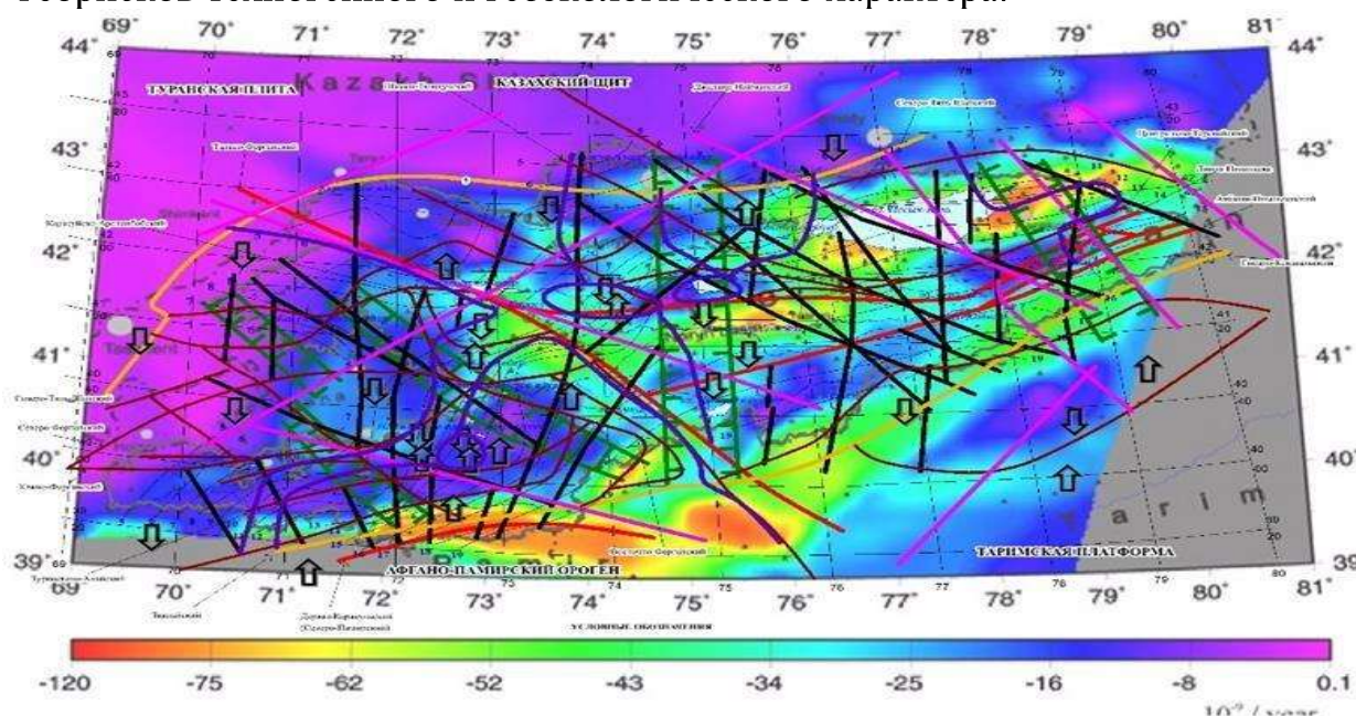
Рисунок. 19. НИГ карта поля скоростей геодформационного сжатия и трансформации палеопрочности полигрантов актуотектоническими движениями, активизирующими в прогностическом отношении геориски от землетрясений и склоновых опасных процессов в земной коре, воздействующие на рудники и карьеры при освоении месторождений полезных ископаемых на территории Кыргызстана и трансграничных районах со странами Центральной Азии
