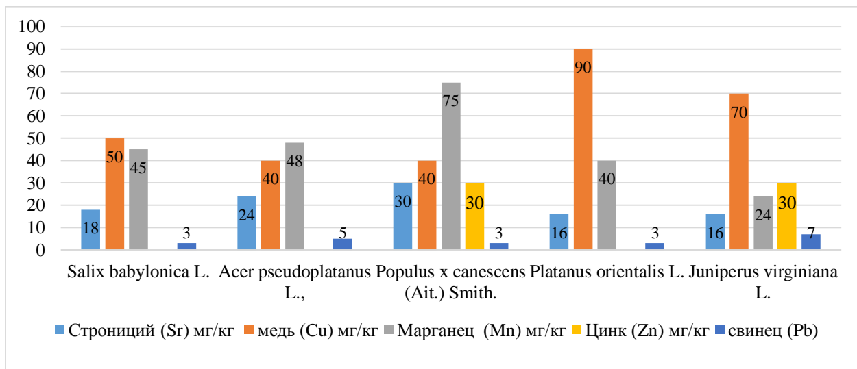
3.3.2.1-сүрөт. Ош шаарындагы дарак өсүмдүктөрүнүн жалбырактарындагы стронций (ВК), жез (вк), марганец (ВК), коргошун (вк) жана цинк (вк) болушунун көрсөткүчтөрү.
