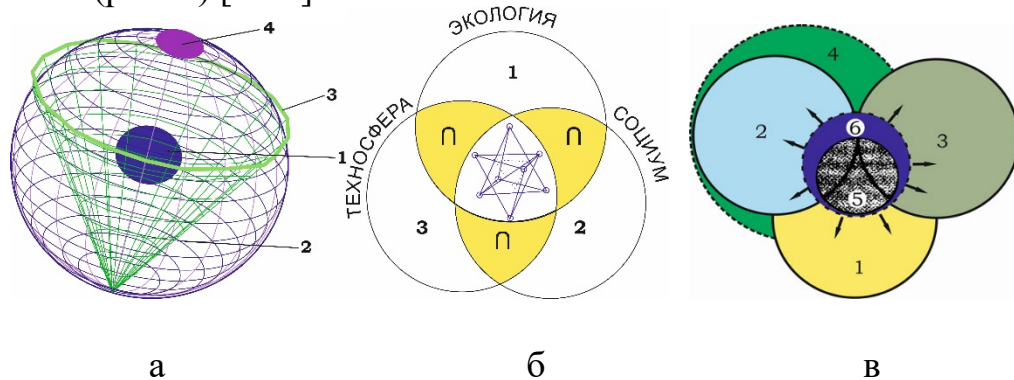
Рисунок 2. Обоснование на базе моделей ноосферы Вернадского В.И. (1935) и Трофимова В.Т., Королева В.А. (2014), разработанного нового научного направления в науках о Земле ноосферной инженерной геологии (НИГ на примере месторождений полезных ископаемых Кыргызского Тянь-Шаня и Памиро-Алая), где: а) Земля - 1; пространство ноосферы - 2; временной конус - 3; информационный банк - 4; б) триадная связь «экологии-социума-техносферы» в цветке ноосферного разума; в) соотношение основных геосфер Земли по Трофимову В.Т. и Королеву В.А.: литосфера - 1; гидросфера - 2; атмосфера - 3; биосфера - 4; ноолитосфера - 5; ноосфера - 6
