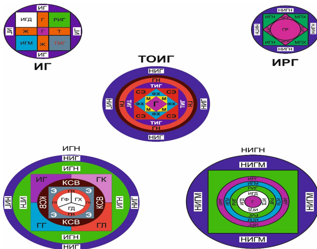
Рисунок 3. Обоснование круговыми диаграммами этапов становления нового научного направления ноосферной инженерной геонимии (НИГН) на примере месторождений полезных ископаемых во взаимосвязи с грунтоведением, инженерной и экологической геологией (ИГ), инженерно-рудничной геологией, технической мелиорацией грунтов, геологической, физико-химической, механико-математической, социально-экономической и основами теории инженерной геологии (ТОИГ), гидрогеологии, геокриологии,
