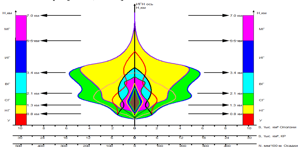
Рисунок 25. Инженерно-геономическая ноосферная модель вертикальной повысотной закономерности распространения, типизации и прогноза георисков от оползней, атмосферных осадков, активизирующихся при освоении полезных ископаемых на территории Кыргызстана.
