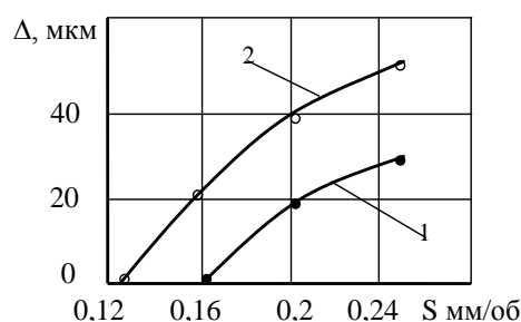
3.14 сүрөт – А1 классындагы жогорку тактыктагы көзөөчтөр менен көзөөдө көзөнөктөрдүн схемасынын берилүү ылдамдыгынан көз карандылыгы: 1 – кесүү ылдамдыгы 4,32 м/мин, 2 – 5,53 м/мин.
