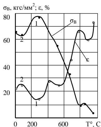
3.6 сүрөт – Конструкциялык болотторду иштетүүдө бекемдиктин жана ийкемдүүлүктүн температурадан көз карандылыгы
