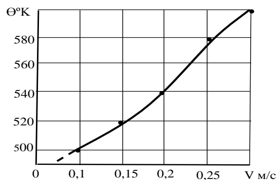
3.8 сүрөт - Структуралык көмүртектуу болотту жогорку ылдамдыктагы болот кескичтер менен токарууда кесүү температурасынын кесүү ылдамдыгына көз карандылыгы
