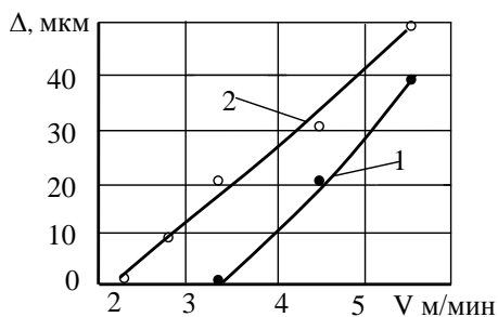
3.15 сүрөт – А1 классындагы жогорку тактыктагы көзөөчтөр менен көзөнөктөрдү көзөө ылдамдыгынан көз карандылыгы: 1 – берүү 0,2 мм/айн, 2 – 0,25 мм/айн.
