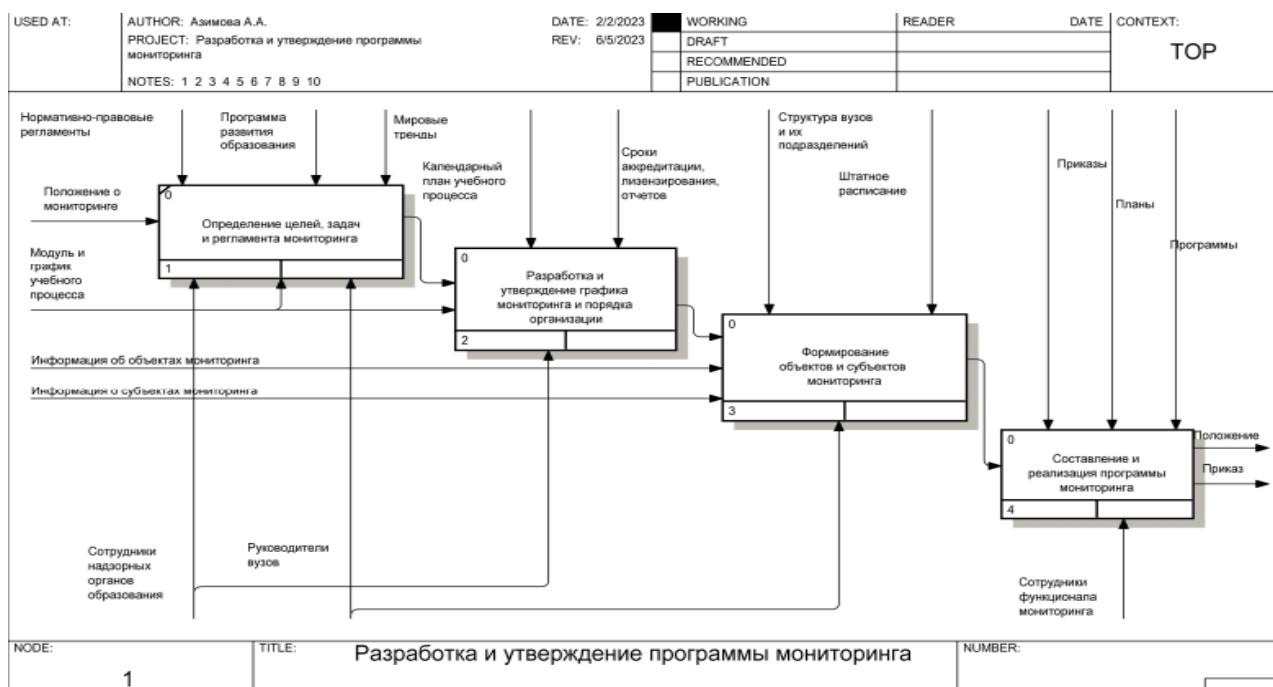
4.5- сүрөт - Мониторинг программасын иштеп чыгуу жана бекитүү процессинин сүрөттөлүшү
