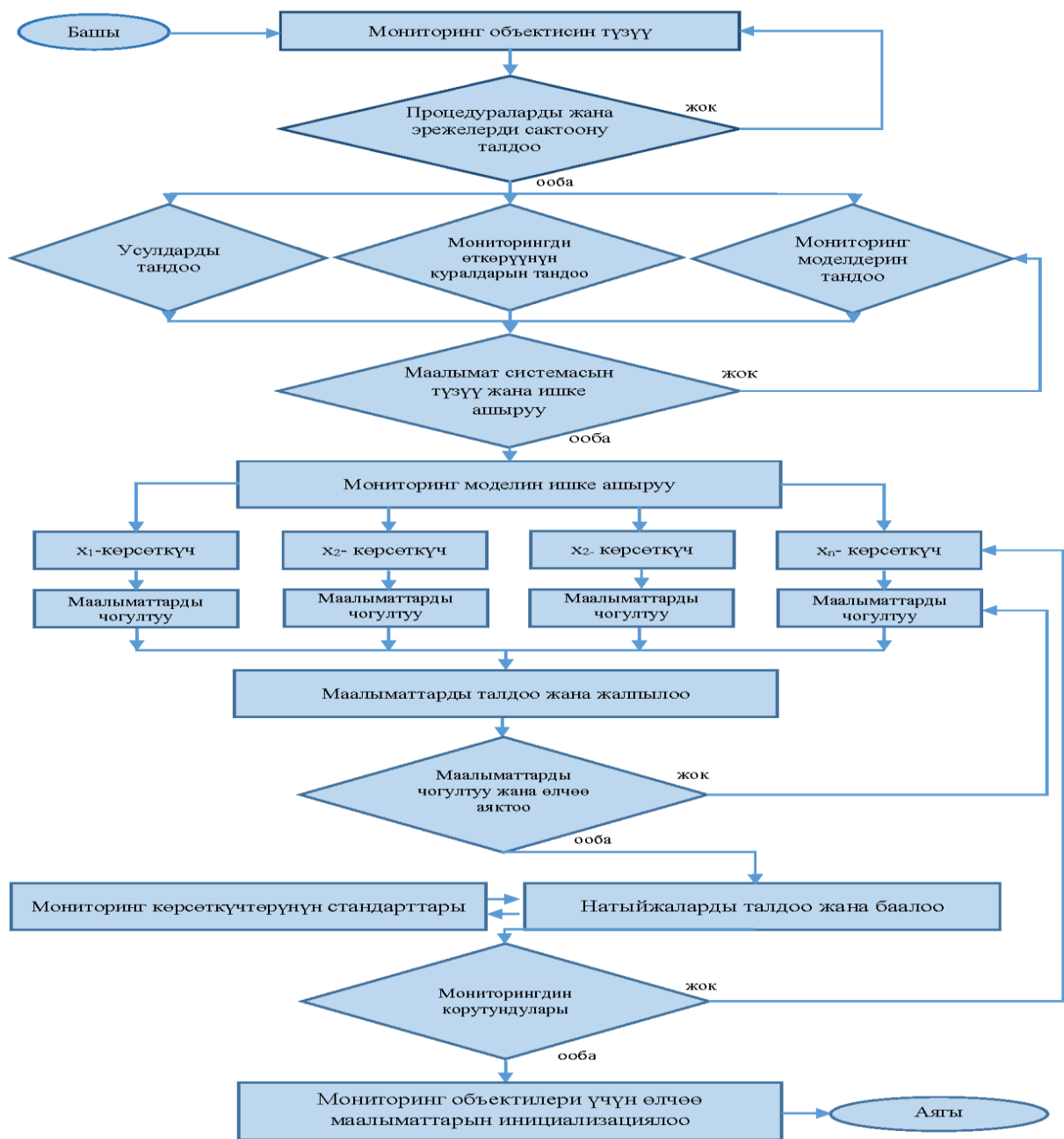
3.7-сүрөт - Билим берүү мониторингинин моделин түзүү алгоритми
