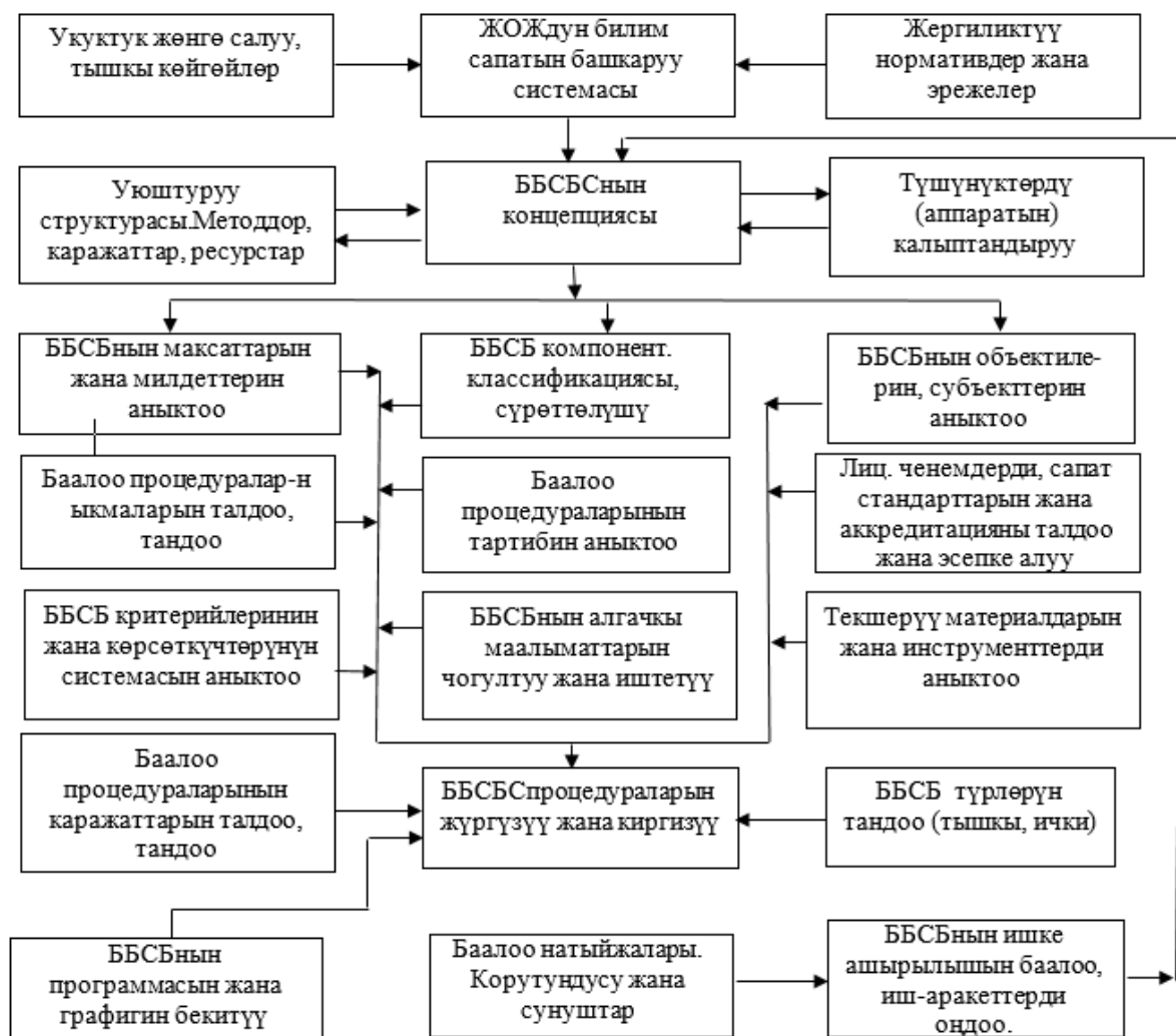
3.6-сүрөт - Билим берүүнүн сапатын баалоо системасын калыптандыруу
