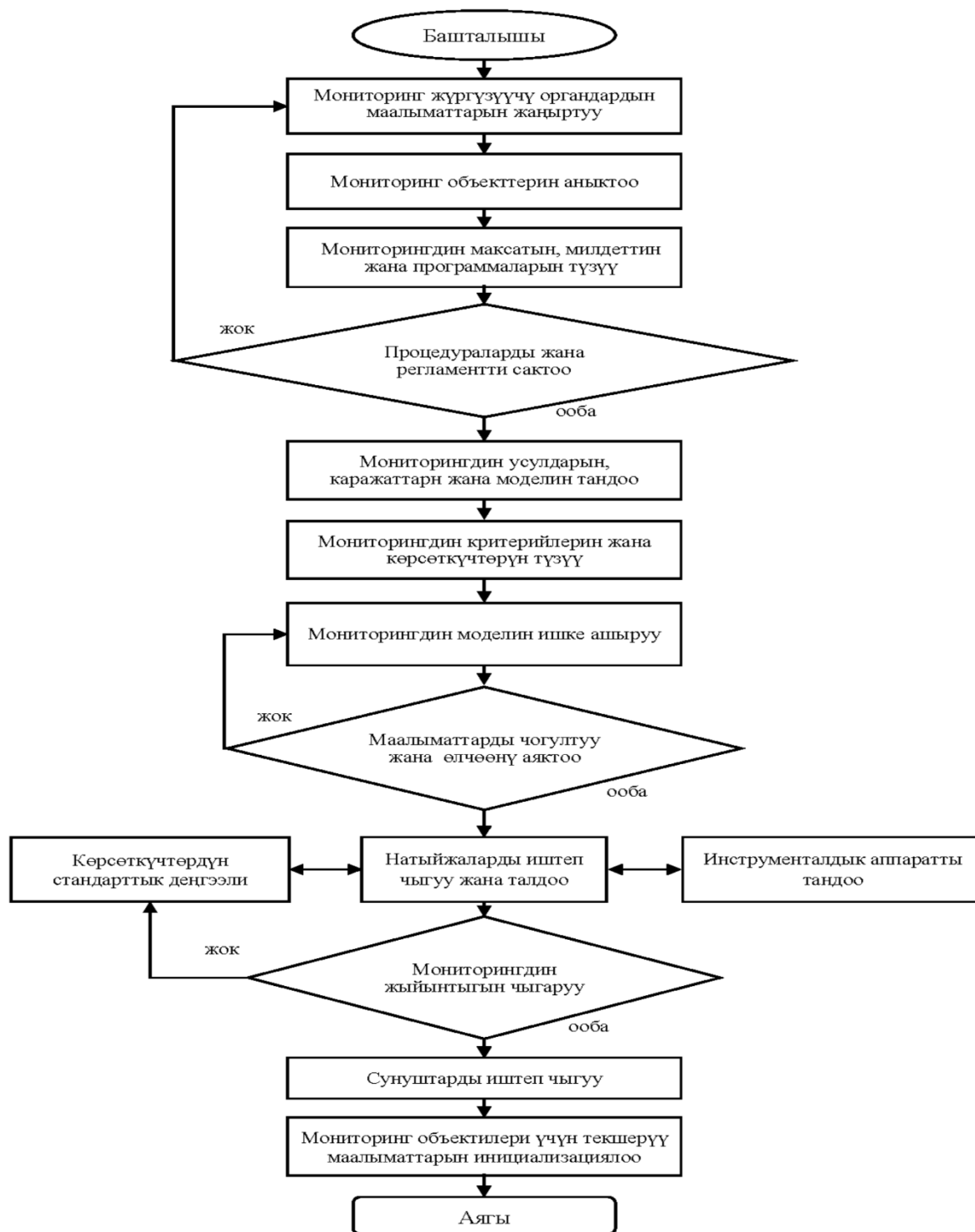
3.4-сүрөт - Билим берүүнүн мониторинг системасын түзүү алгоритми
