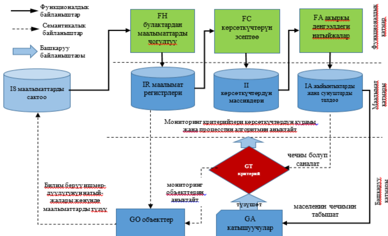
4.1-сүрөт - Билим берүү мониторинг системасынын концептуалдык модели
