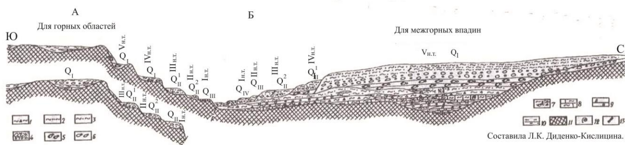
Рисунок 2.1.2 - Схема взаимоотношений кайнозойских отложений в Северной Джунгарии (по Диденко-Кислицыной, 2006).
