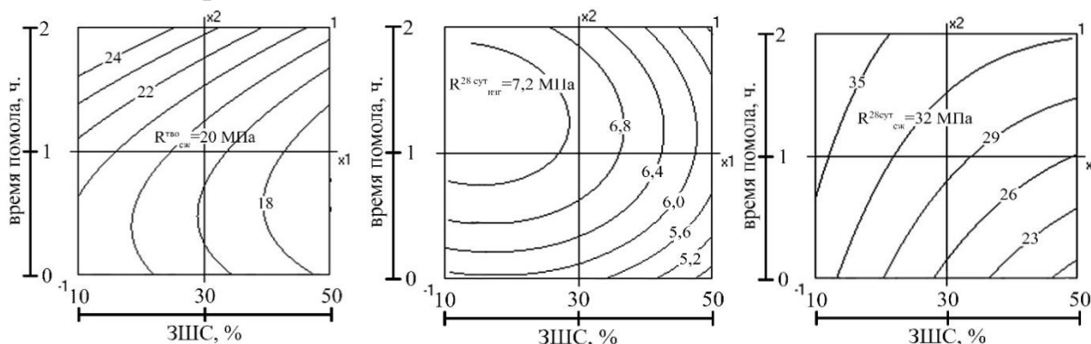
Рисунок 2 - Прочность после ТВО ( R^{\text{ТВО}}_{\text{сж}} ), при 28 сутках изгиб ( R^{28\text{сут}}_{\text{изг}} ), сжатие ( R^{28\text{сут}}_{\text{сж}} ) образцов цементнозолошлакового вяжущего ЦЗШВ
