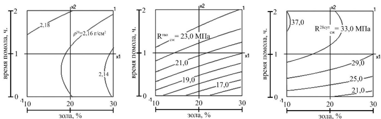
Рисунок 1 - Плотность ( \rho^{28} ), прочность после ТВО ( R^{\text{ТВО}}_{\text{сж}} ) и при 28 сутках ( R^{28\text{сут}}_{\text{сж}} ) образцов цементнозольного вяжущего ЦЗВ
