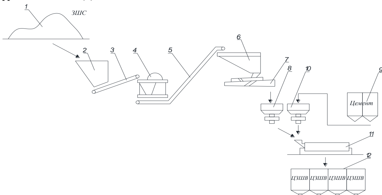
Рисунок 8 - Технологическая схема производства цементнозолошлаковых вяжущих веществ: 1-ЗШС; 2,6 - приемный бункер; 3,5 - ленточный транспортер; 4 - Щековая дробилка; 7 - грохот; 8, 10 - бункер с питателем для цемента и золошлаковой смеси; 9 - силосы для цемента; 11 - шаровая мельница; 12 - силосы для золошлакоцементных композиционных вяжущих веществ (ЦЗШВ)
