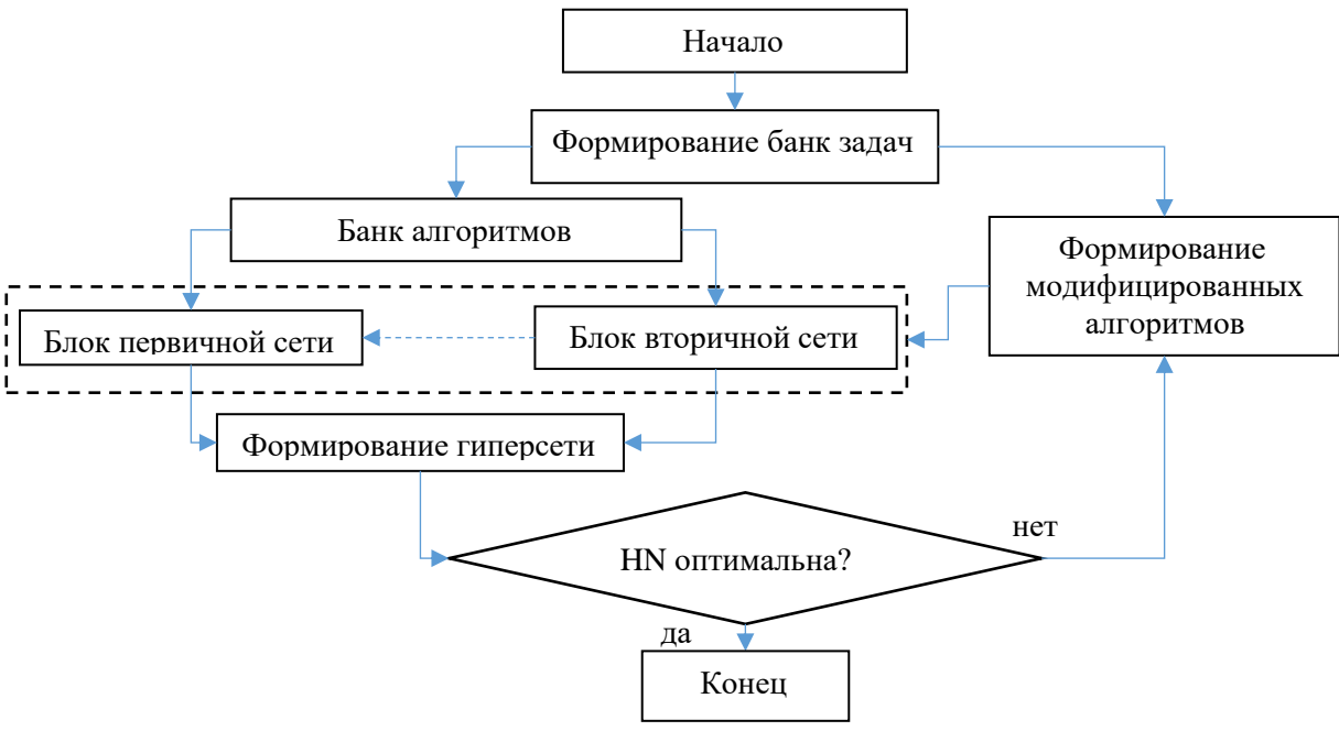
Рисунок 10 – Представление методов оптимизации в виде блок-схемы
