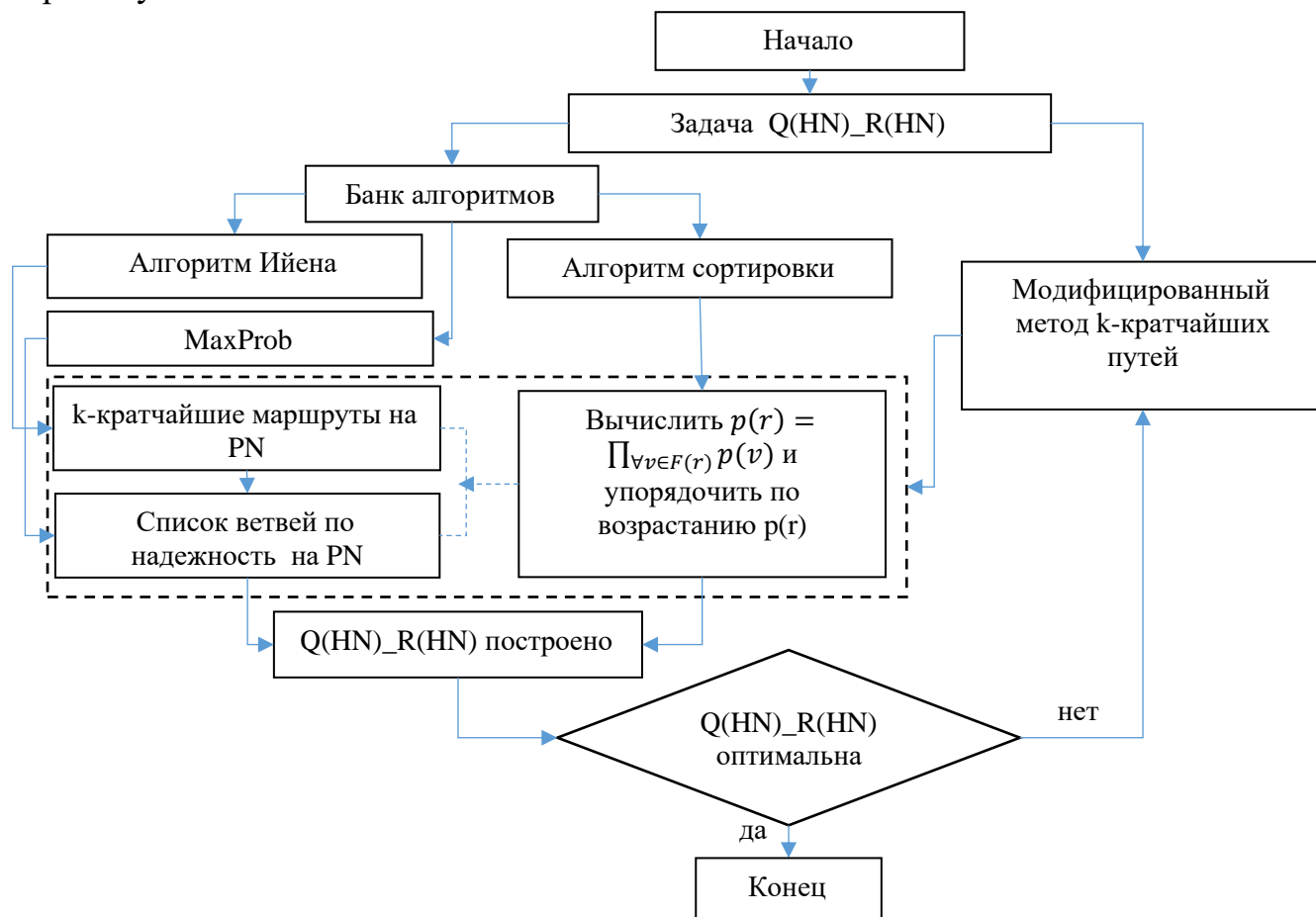
Рисунок 15 – Блок-схема модифицированного метода k-кратчайших путей
