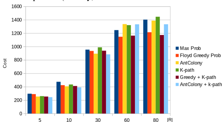
Рисунок 16 – Результаты работы алгоритмов для решетки 10×10, количество ребер вторичной сети от 5 до 80
