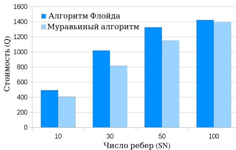
Рисунок 14 – Численные результаты: стоимость для решетки 10x10, для количества ребер от 10 до 100
