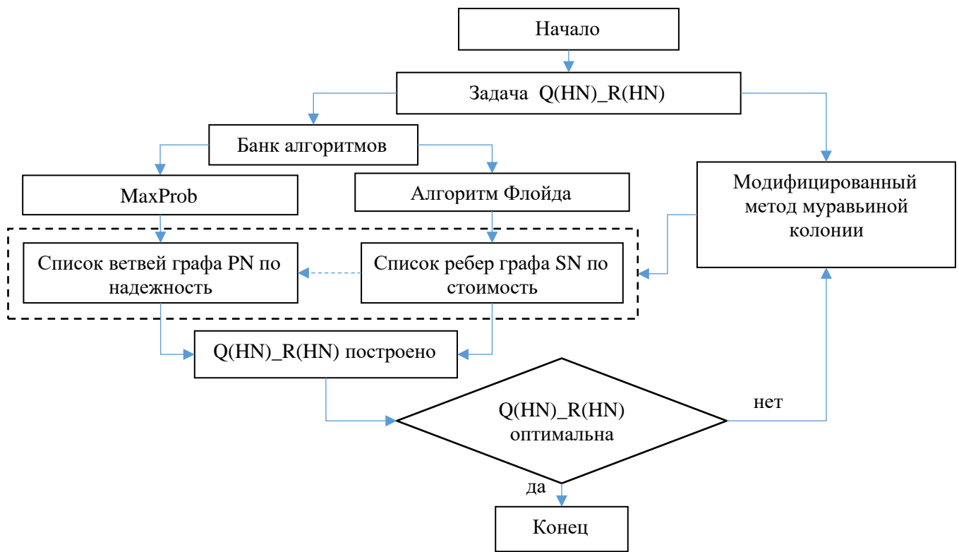
Рисунок 13 – Представление модифицированного AntColony в виде блок-схемы
