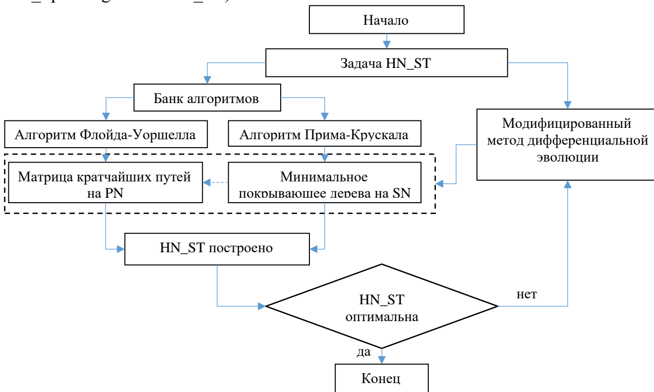
Рисунок 11 – Представление ММДЭ в виде блок-схемы
