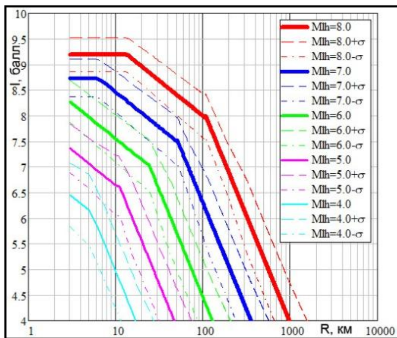
Рисунок 4.2.1 - Зависимость сейсмической интенсивности от расстояния до источника с магнитудой M_{LH} для землетрясений со взбросовой кинематикой подвижки в очаге землетрясения. Графики построены С.А. Перетокиным (НП ЭЦ РОПР) по данным Ф.Ф. Аптикаева (ИФЗ РАН) [12].
