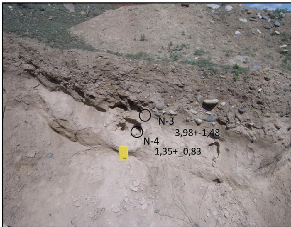
3.1.2.8 - сүрөт. Геологиялык катмарлардын жашын аныктоо үчүн OSL үлгүлөрүн алуу жерлери жана алардын натыйжалары, Ага Хан университетинин тилкеси, Нарын шаарынын батыш тарабы.
