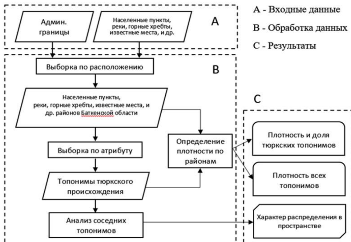
Рис. 2. Алгоритм географического анализа тюркоязычной топонимии* *составлено автором
