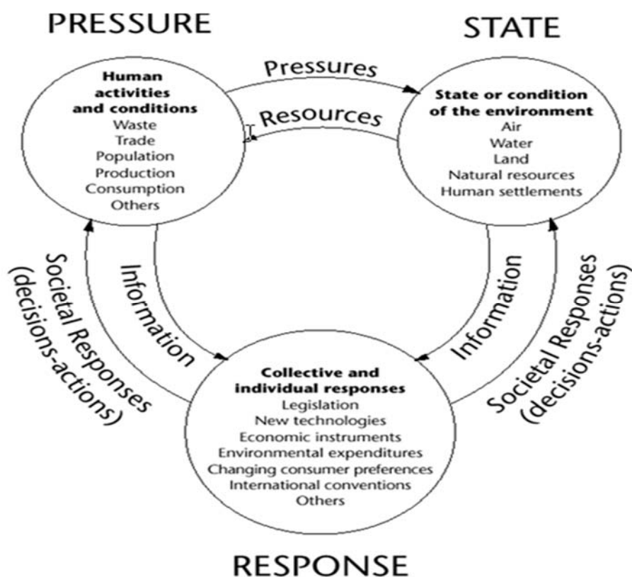
Рисунок 1.2.1 Схема взаимосвязи компонентов PSIR (источник: G. Braathen, 2015)
