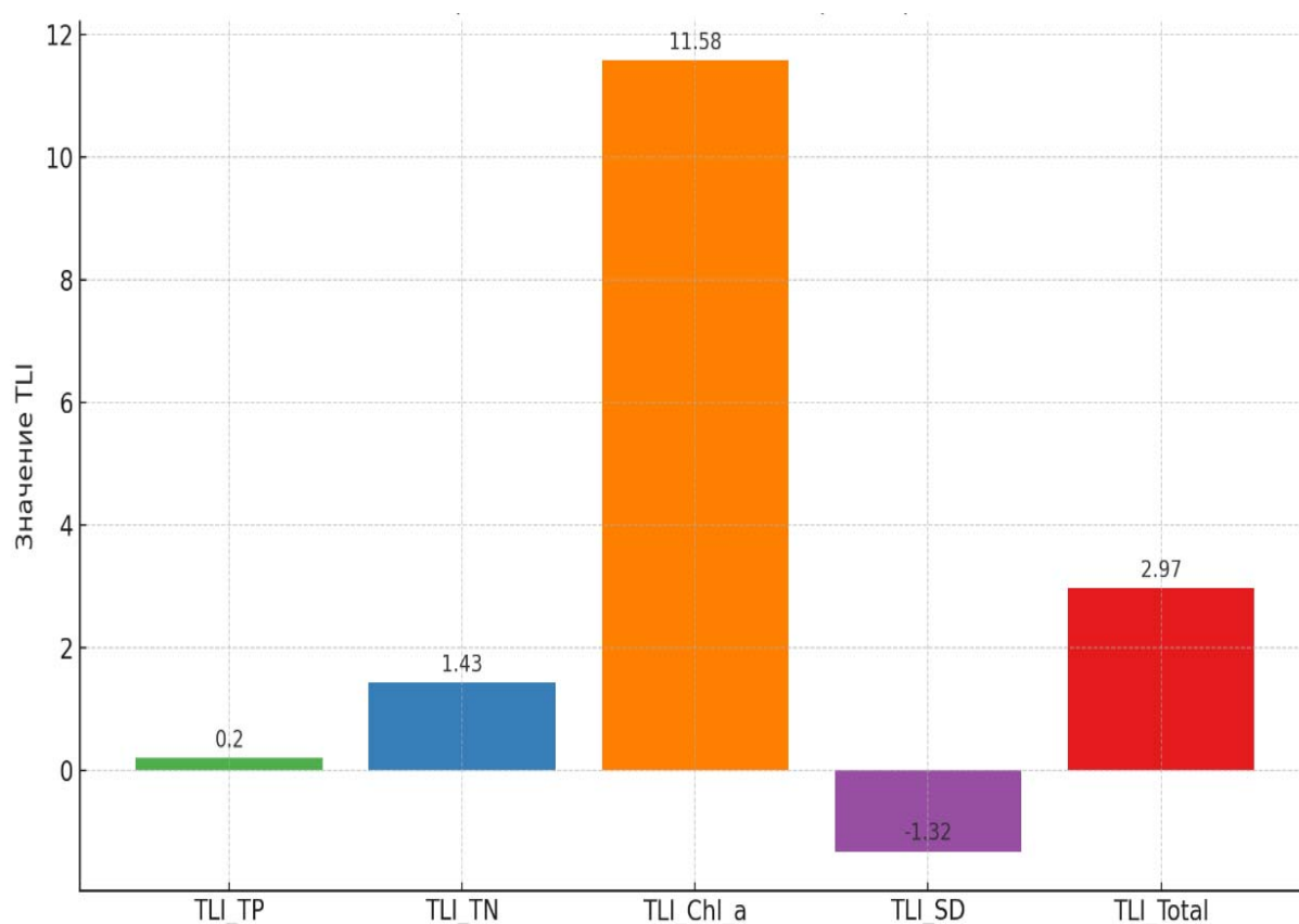
Рисунок 4.2.4 Трофический индекс (TLI): средние значения по основным параметрам.
