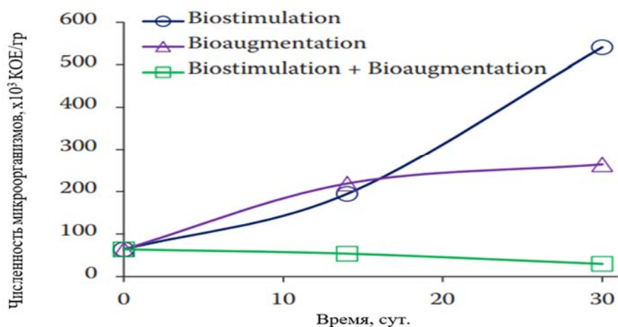
Рисунок 5.1.3. Динамика численности бактерий в нефтезагрязнённой почве в процессе биоремедиации
