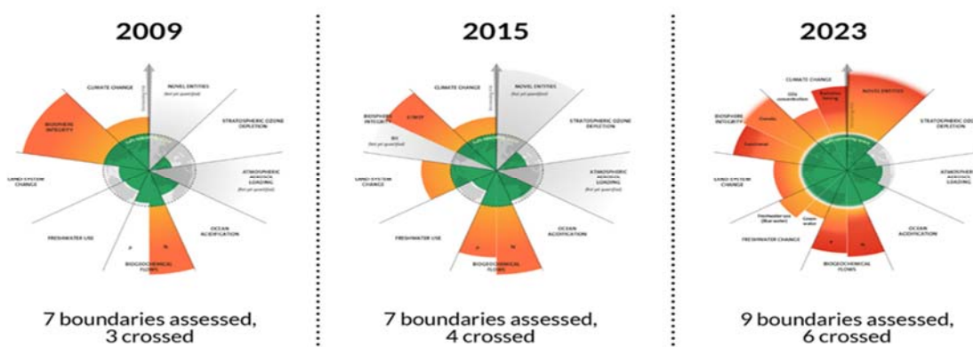
Рисунок 1.1.5 Эволюция системы планетарных границ. Лицензировано CC BY-NC-ND 3.0 (Credit: Azote for Stockholm Resilience Centre, Stockholm University. Основано на материалах Richardson et al. 2023, Steffen et al. 2015 и Rockström et al. 2009)
