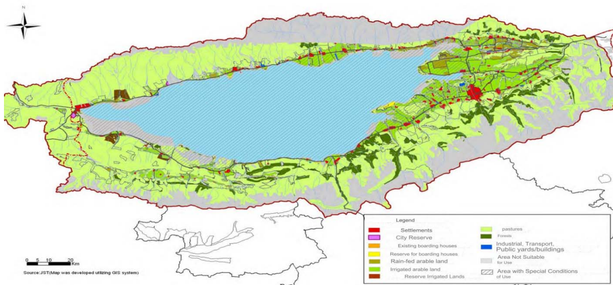
Рисунок 4.6.2 Землепользование в Иссык-Кульской области
