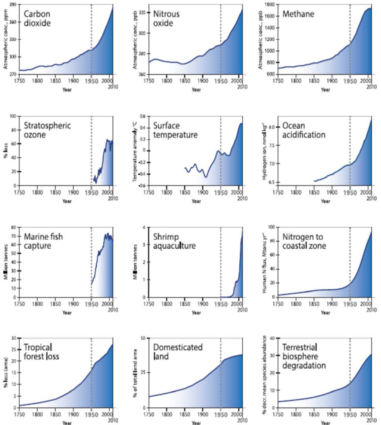
Рисунок 1.1.2 Тенденции изменения показателей структуры и функционирования системы Земли с 1750 по 2010 год (источник: Steffen, Broadgate et al., 2015)
