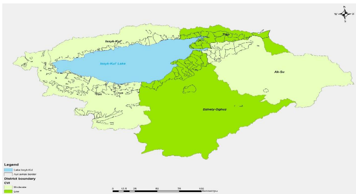
Рисунок 4.6.5. Пространственная изменчивость индекса уязвимости побережья (CVI) оз.Иссык-Куль
