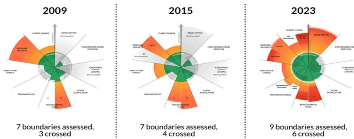
Рисунок 1.1.6 Эволюция системы планетарных границ. Лицензировано CC BY-NC-ND 3.0 (Credit: Azote for Stockholm Resilience Centre, Stockholm University. Основано на материалах Richardson et al. 2023, Steffen et al. 2015 и Rockström et al. 2009)
