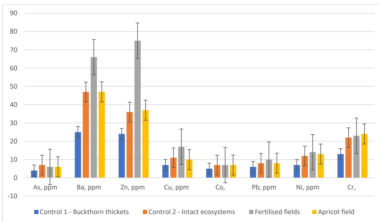
Рисунок 4.4.2 Содержание тяжелых металлов в исследуемых образцах почв
