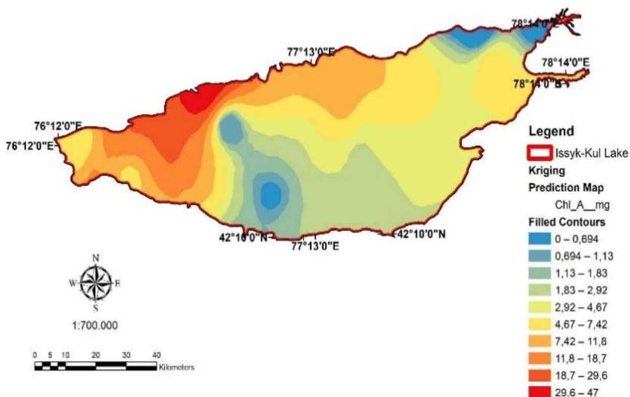
Рисунок 4.2.9 Пространственное распределение концентраций Chl-a
