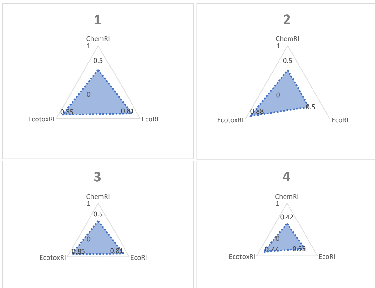
Рисунок 3.2.4 Рассчитанные индексы риска (RI): химический (ChemRI), экотоксикологический (EcotoxRI), экологический (EcoRI); количество хвостов 1-4; площадь темного треугольника отражает степень нарушения почвы.
