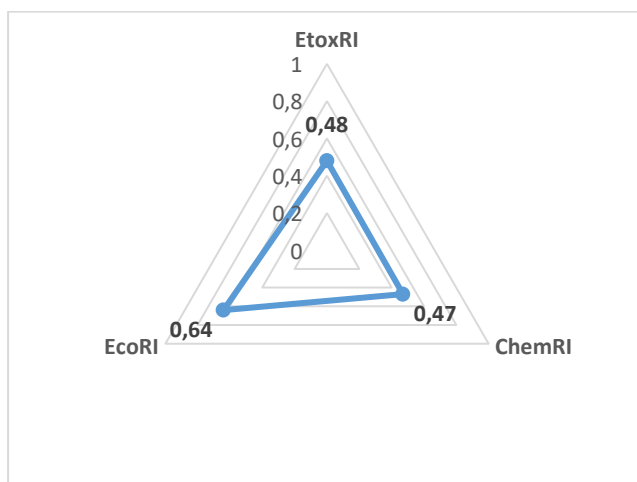
Рисунок 3.2.2 Рассчитанные индексы риска (RI): химический (ChemRI), экотоксикологический (EcotoxRI), экологический (EcoRI)
