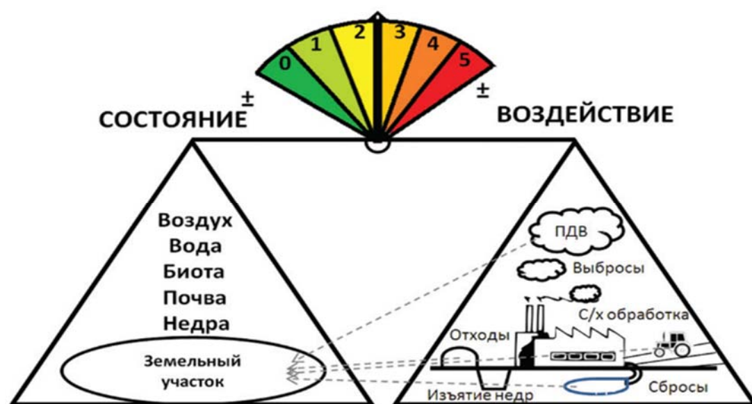
Рисунок 3.1.1 Схема экологического равновесия в системе “состояние – воздействие” источник А.Яковлев, 2019)
