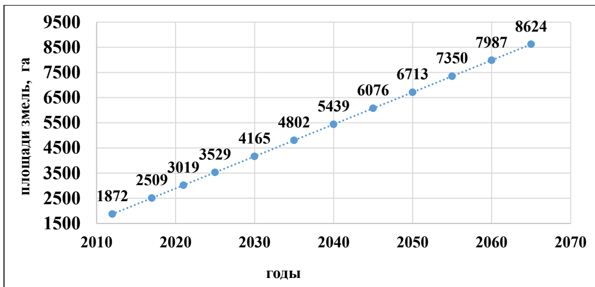
Рисунок 4.3.3 Прогноз преобразования ПБЗ при нынешней тенденции преобразования ПБЗ
