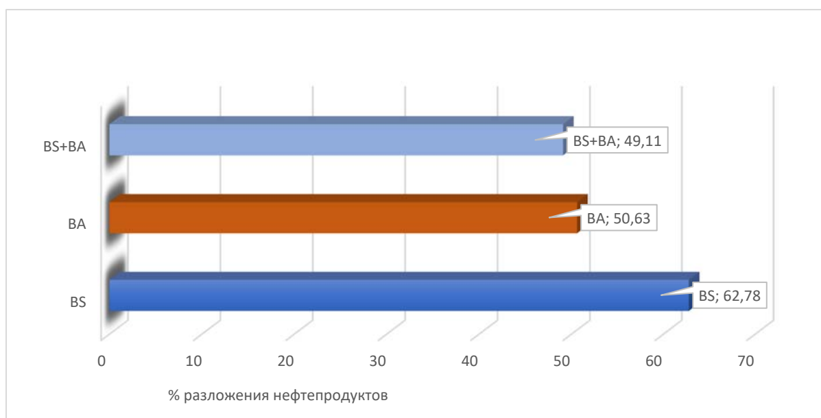
Рисунок 5.1.1 Рисунок 1. Разложение нефтепродуктов после 90 дней опыта, %. BS - биостимуляция; BA – биоаугментация
