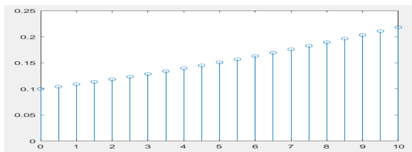
Рисунок 1. Коэффициент роста равен e=0,1
