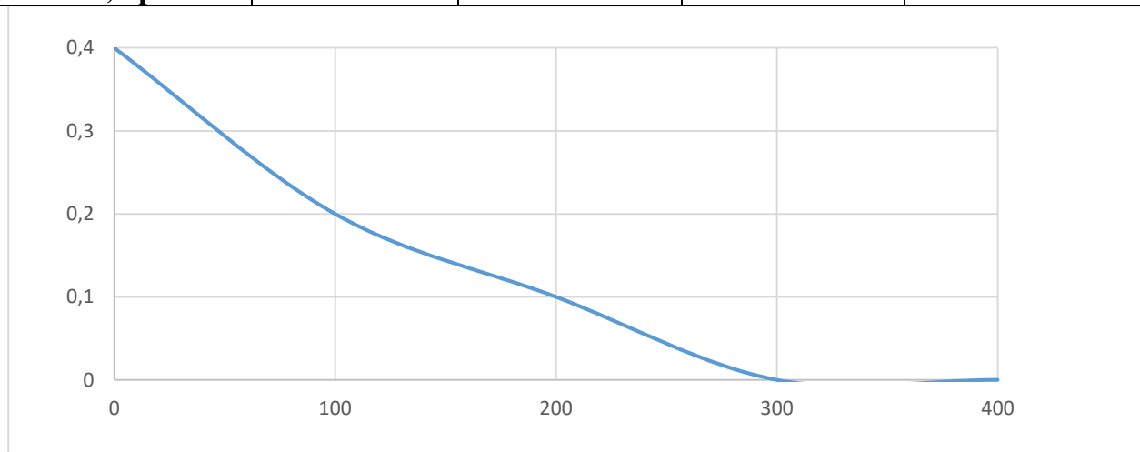
Рисунок 17. Итоговая зависимость коэффициента роста кустарника карагана от концентрации применяемого гербицида
