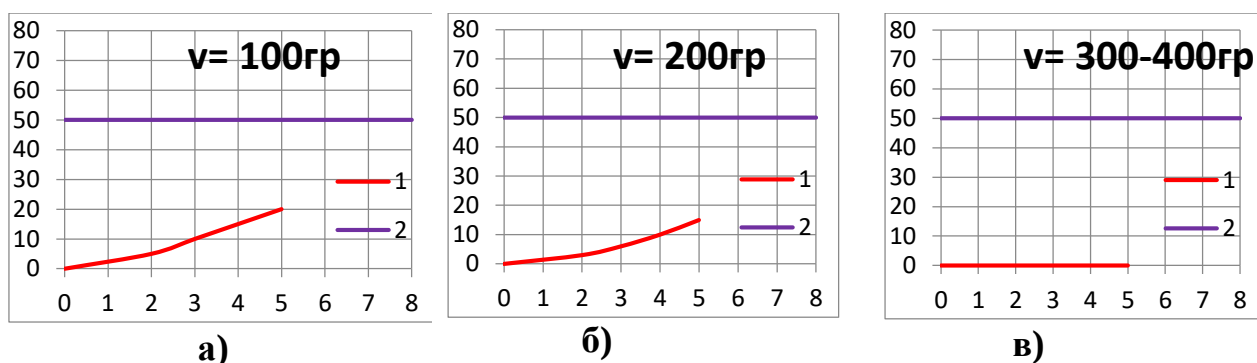
Рисунок 11. Зависимость жизнеспособности кустарника карагана в течение 5 лет после воздействия гербицида концентрации а) 100г/10л, б) 200г/10л, в) 300-400г/10л:
