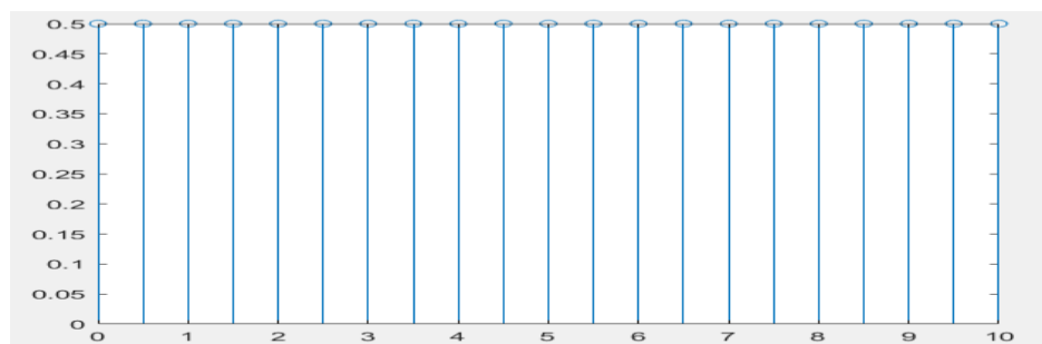
Рисунок 3. Коэффициент роста равен \epsilon=0,0
