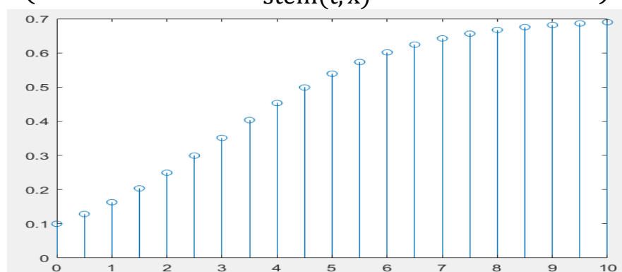
Рисунок 2. Коэффициент роста равен e=0,6
