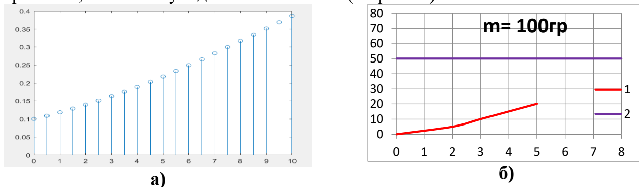
Рисунок 14. Сравнение результатов математической модели Ферхюльста в программе MATLAB R20176 а) с результатами эксперимента б) при воздействии гербицида концентрации 10 г/л
