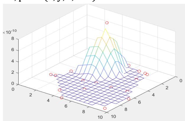
Рисунок 4. Занимающая площадь через 10 лет
