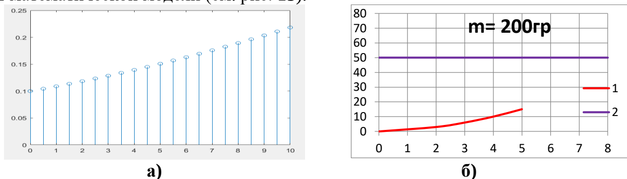
Рисунок 15. Сравнение результатов математической модели Ферхюльста в программе MATLAB R20176 а) с результатами эксперимента б) при воздействии гербицида концентрации 20 г/л
