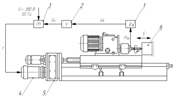
Рис. 2. Принципиальная схема системы автоматического управления скоростью электродвигателя
