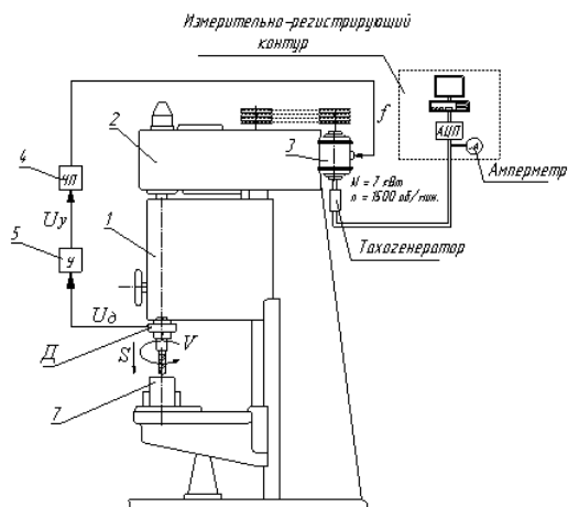
Рис.11 Схема стенда для исследования силы резания при сверлении преобразователя частоты тока 4; специальной, ступенчатой заготовки 7; тахометра и измерительно-регистрирующего комплекса.
