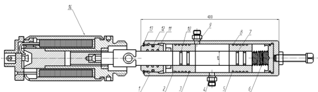
Рис. 7. Конструкция регулятора расхода жидкости
