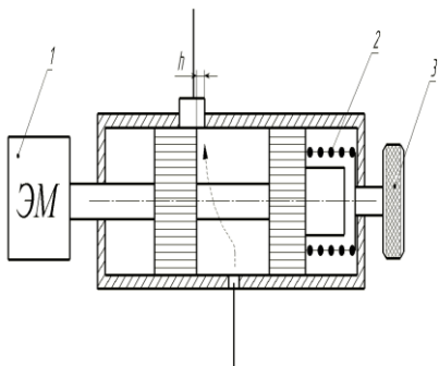
Рис. 5 Схема конструкции регулятора расхода жидкости ЭМР-8
