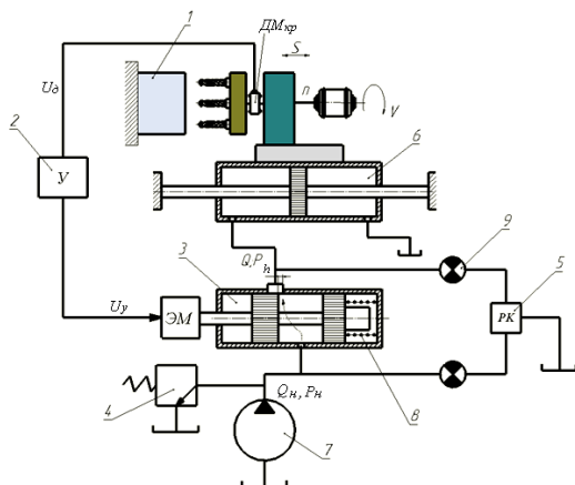
Рис. 1. Принципиальная схема системы автоматического управления подачей гидравлической силовой головки
