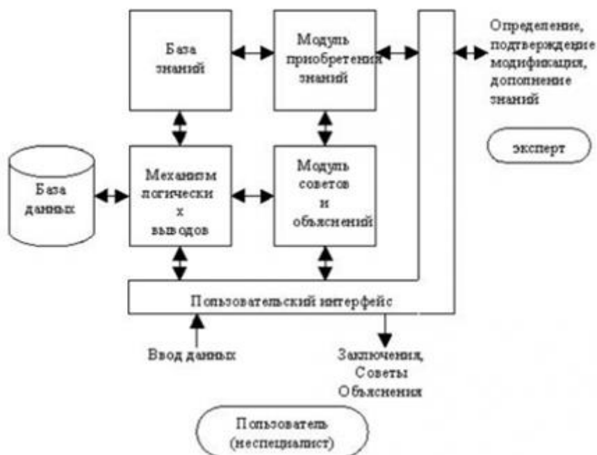
1 - сүрөт- Модель экспертной системы
