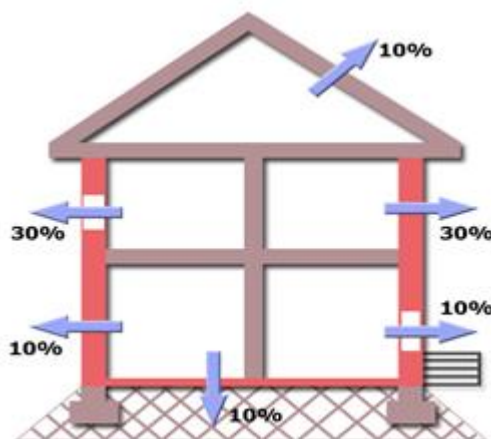
3- сүрөт - Имараттан жылуулук жоготууларынын схемасы.
