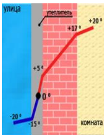
4 - сүрөт – Дубалдарды сырттан жылуулоо
