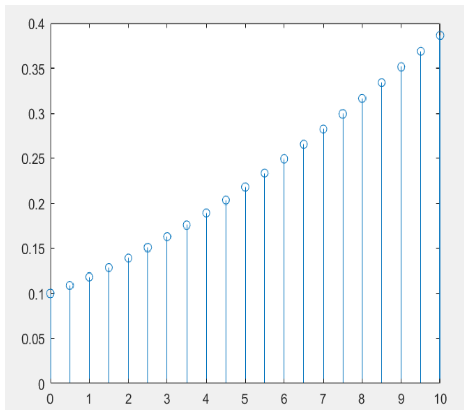
3.5.1-сүрөт. а) MATLAB R20176 программасындагы Ферхюльста математикалык моделдинин жыйынтыктарын б) гербициддин 10 г/л концентрациясындагы эксперименттин натыйжалары менен салыштыруу
