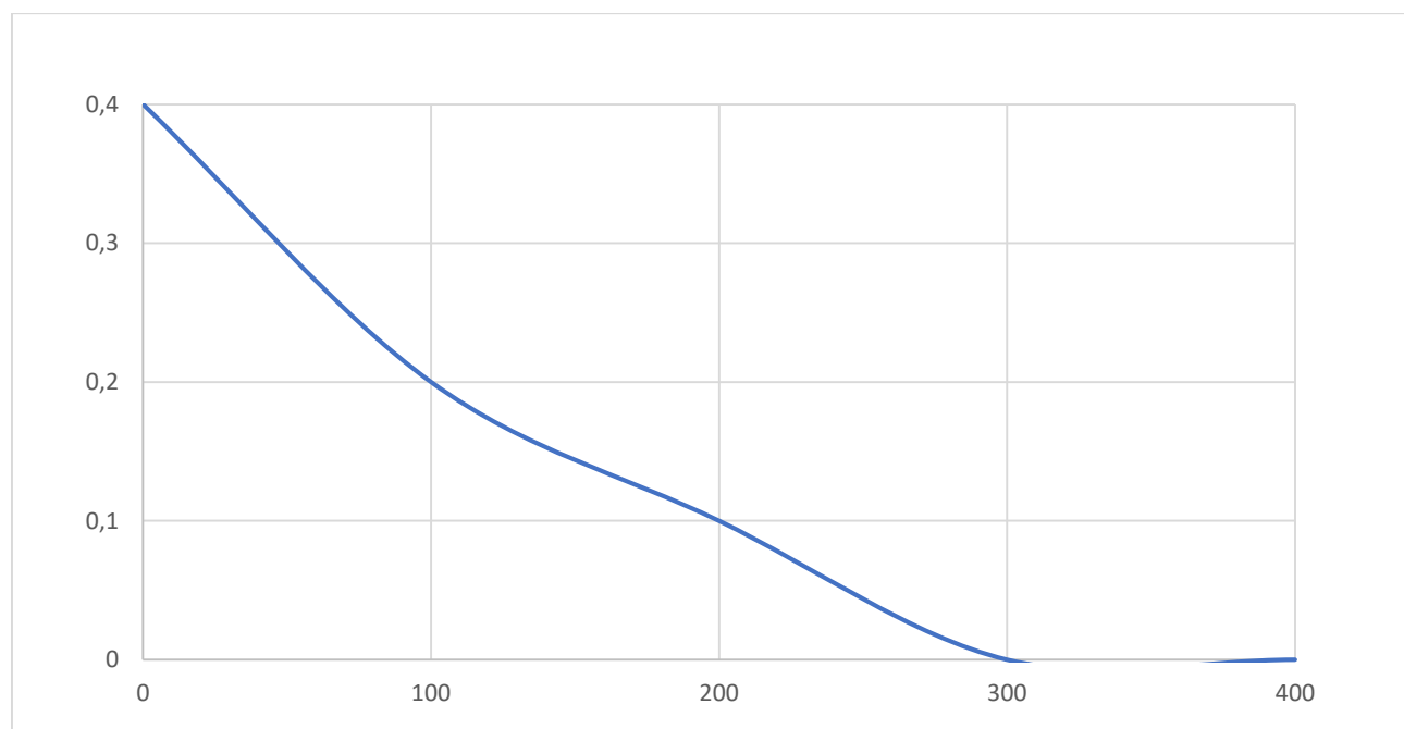
3.5.4-сүрөт. Өсүү коэффициенті менен гербициддин өлчөмүнөн көз карандылыгы
