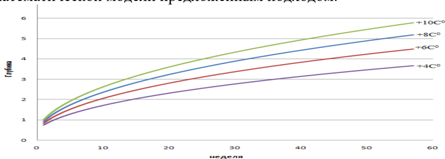
Рис. 3.3 Глубина таяния основание хвостохранилища в зависимости температуры воды.
