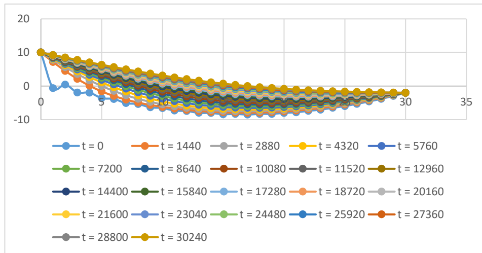
Рис.4.3 Значения температуры в разные моменты времени по глубине
