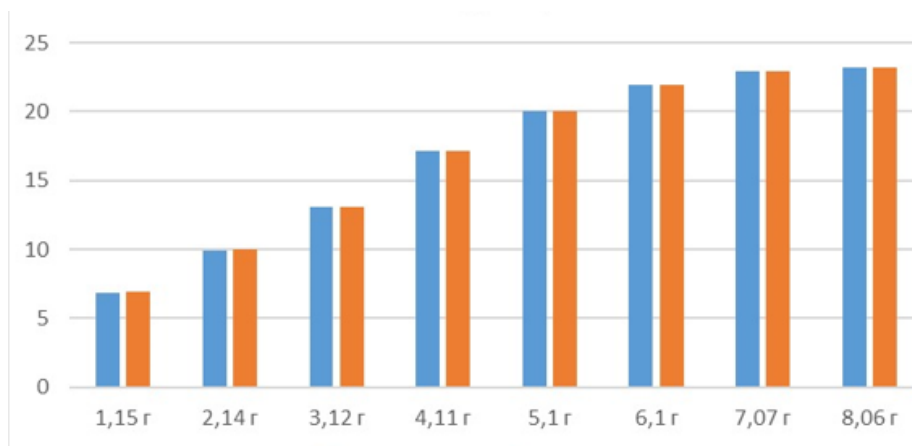
Рис.4.7 Положение нулевой изотермы с учетом и без учета теплообмена
