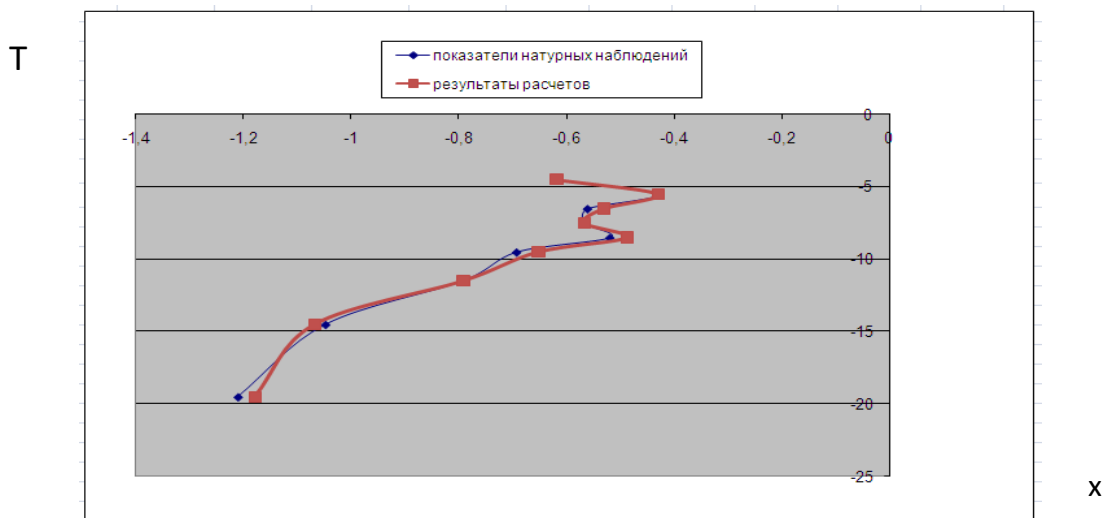
Рис.3.2 Температура грунта
