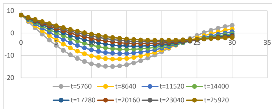
Рис. 4.5 Значения температуры грунта в разные моменты времени в случае, когда на нижней границе принимается граничное условие третьего рода
