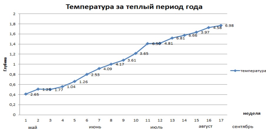
Рис. 3.4. Глубина таяние вечной мерзлоты за теплый период года.
