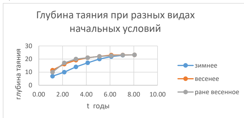
Рис. 4.10 Глубина таяния при разных видах начальных условий
