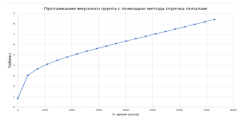
Рис.4.12 Глубина таяния как местоположение нулевой изотермы
