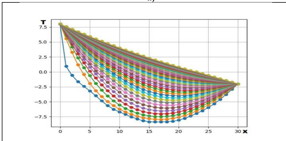
Рис.4.2. Значения температуры грунта под основанием водоема в различные моменты времени
