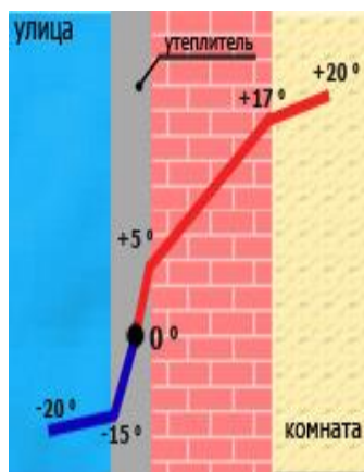
Рисунок 4 - Утепление стен выполнено снаружи помещения
