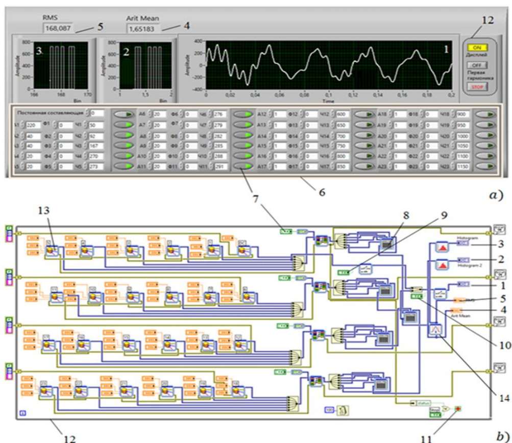
Рисунок 6 - Лицевая панель - а и блок-диаграмма б ВП
