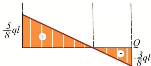
Рисунок 3.3.10.е – Эпюра внутренних напряжений.
