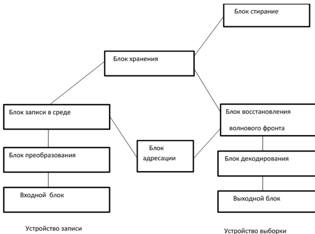
Рис. 2. Набор блоков в ГЗУ.
