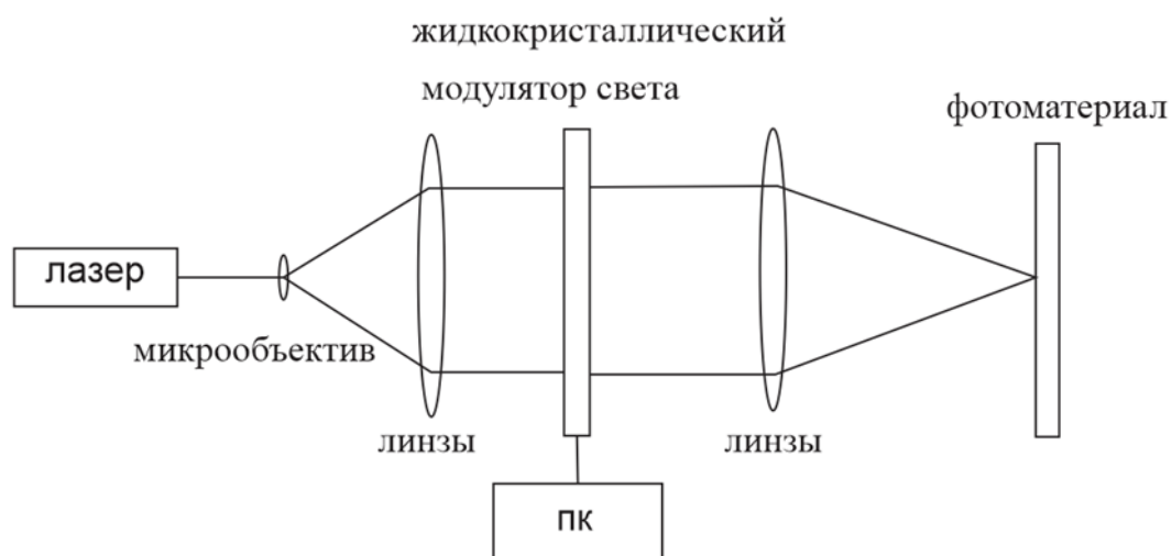
Рисунок 4. Схема записи цифровой информации в виде синтезированных голограмм.
