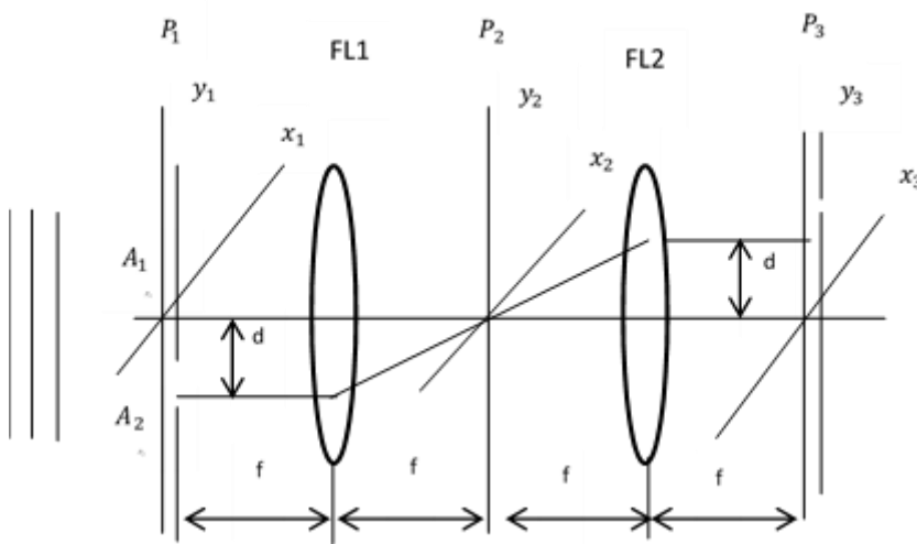
Рисунок 9. Архитектура коррелятора совместного преобразования.
