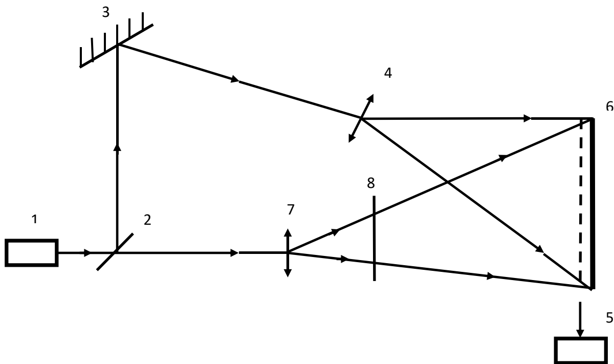
Рисунок 12. Устройство для записи информации на ТП носитель в ИК диапазоне
