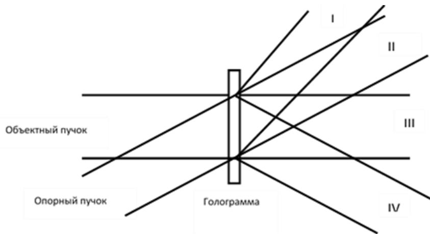
Рисунок 8. Составляющие волнового фронта, восстановленного одновременно опорным и измененным объектным пучка
