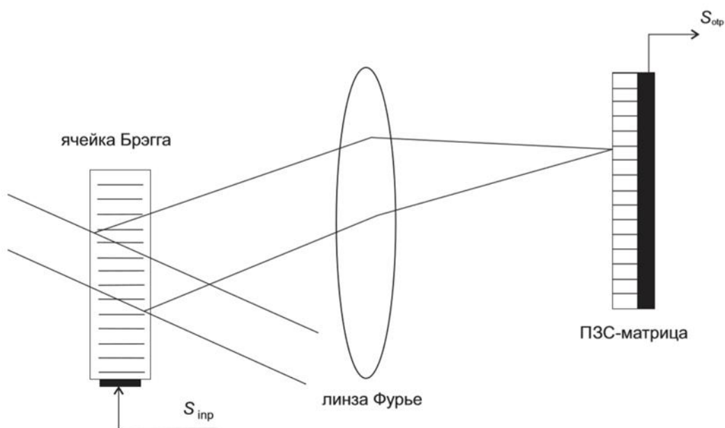
Рисунок 5. Схематическое изображение АОСА с пространственной интеграцией
