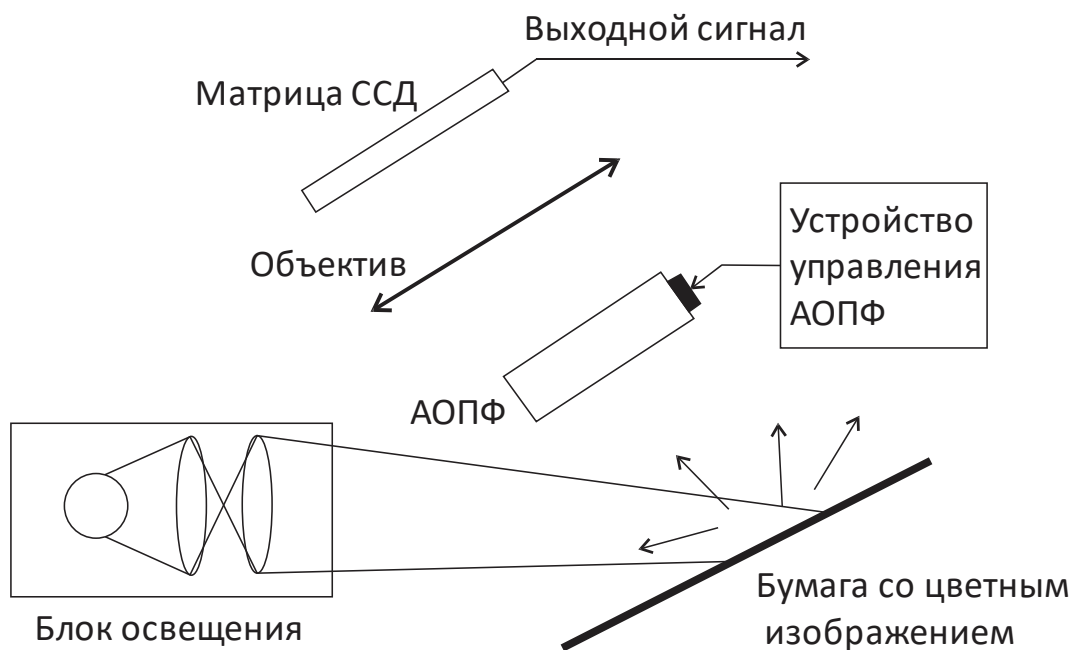
Рисунок 11. Оптическая конфигурация фона бумаги и спектрального состава знаков с использованием АОПФ.
