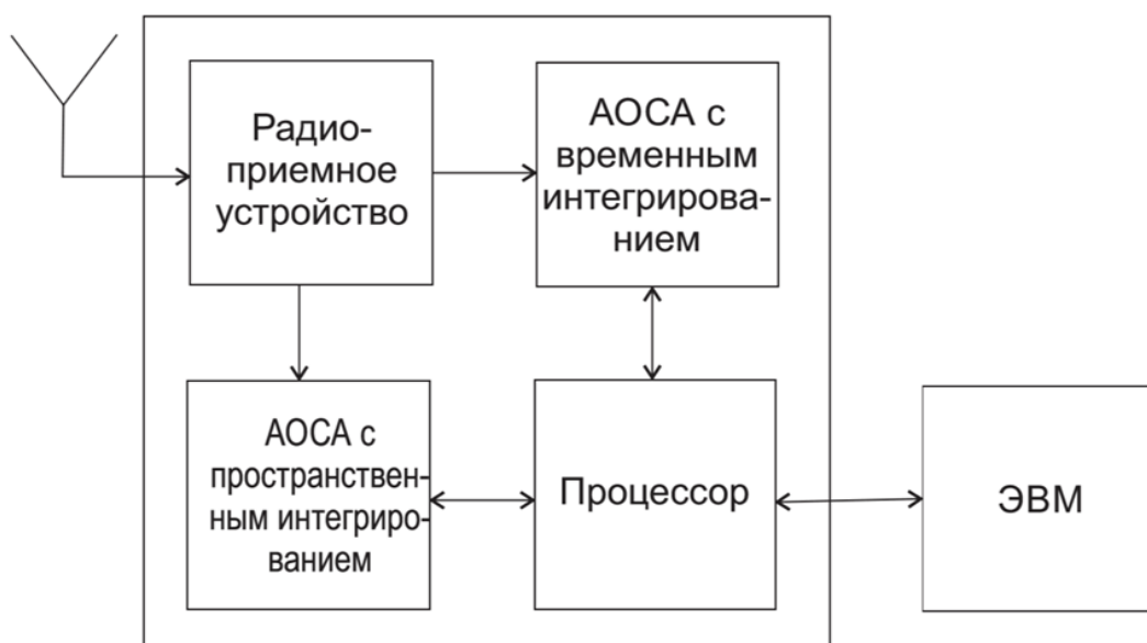
Рисунок 7. Схематическое изображение системы анализа спектра радиочастотного сигнала с отдельными АОСА с временной и пространственной интеграцией, работающими параллельно
