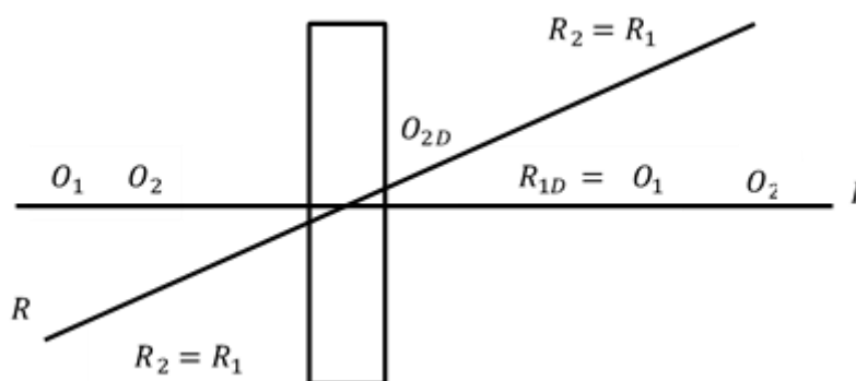
Рисунок 10. Схема двухпучкового восстановления волнового фронта с объемной голограммы.
