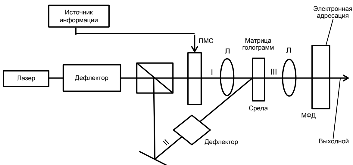
Рисунок 1. Блок-схема голографической памяти
