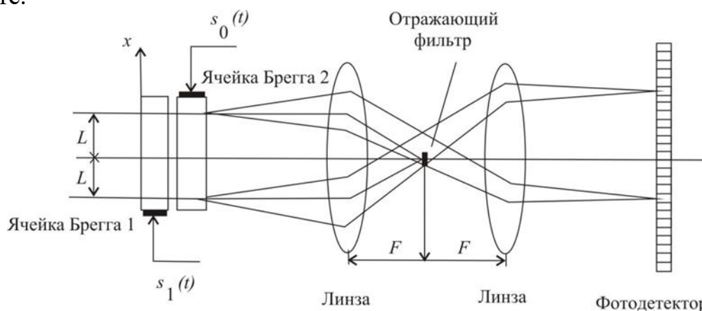
Рисунок 6. Схематическое изображение акустооптического коррелятора с встречно-ориентированными ячейками Брэгга как основы анализатора спектра с интеграцией по времени
