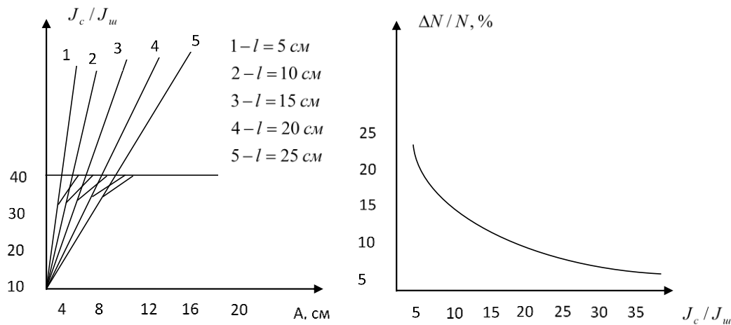
Сүрөт. 5. J_c / J_u (A) жана \Delta N / N (A) көз карандылыктары
