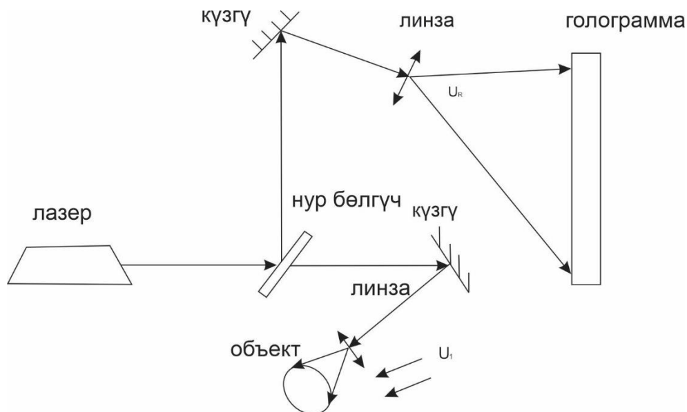
Сүрөт.1. Голографиялык интерферометрияны жазуу үчүн огуна тышкары схема. U_R - таяныч нуру; U_1 - объект нуру.
