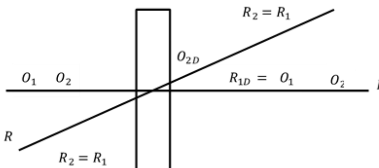
14-сүрөт. Көлөмдүк голограммадан толкун фронтунун эки нурлуу реконструкциясынын схемасы.
