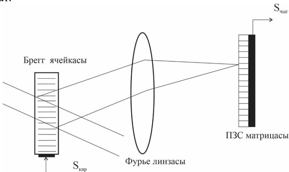
5-сүрөт. АОКАнын мейкиндик интеграциясы менен схемалык чагылдырылышы
