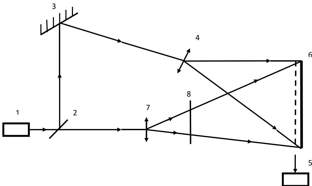
12-Сүрөт. ТПлык материалга маалыматты ИК диапазонунда жазуу үчүн түзүлүш
