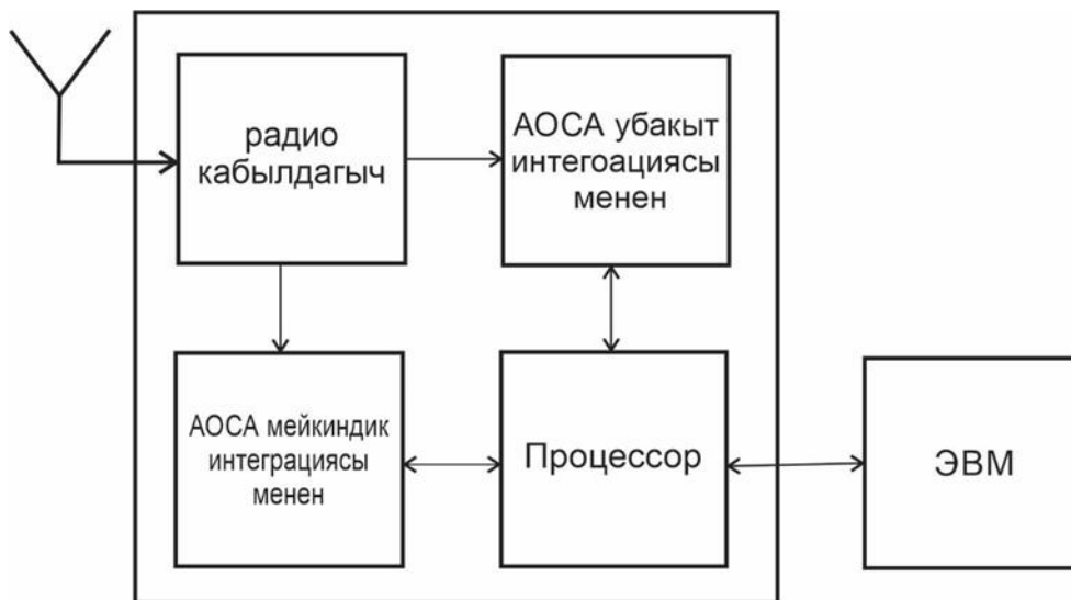
7-сүрөт. Параллель иштеген убакыт жана мейкиндик интеграциясы менен өзүнчө АОСА менен радио жыштык сигналы үчүн спектрдик анализ системасынын схемалык көрүнүшү
