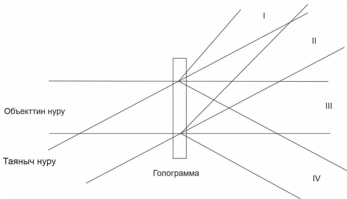
8-сүрөт. Бир эле убакта таяныч жана өзгөрүлгөн объектик нурлары менен реконструкцияланган толкундун фронтунун компоненттери
