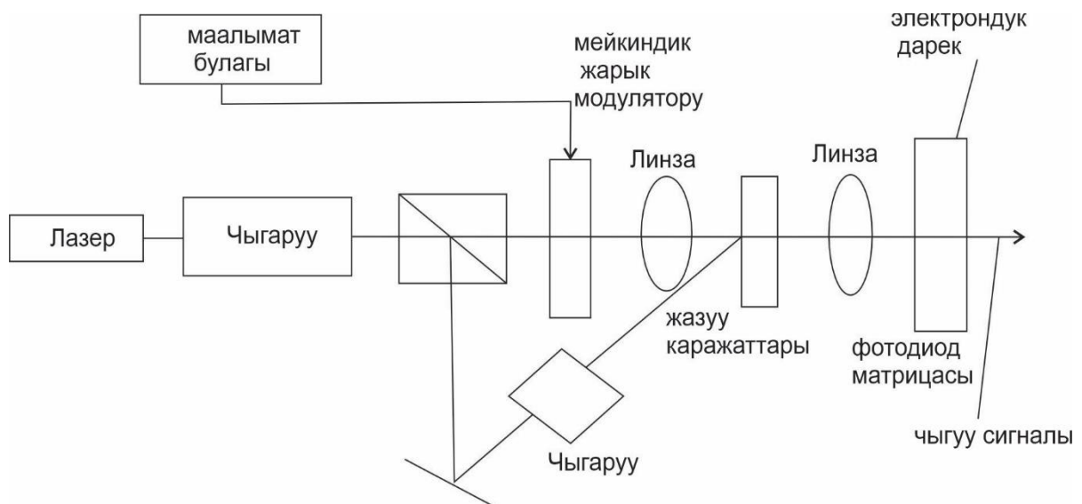
1-сүрөт . Голографиялык эс тутумдун блок – диаграммасы
