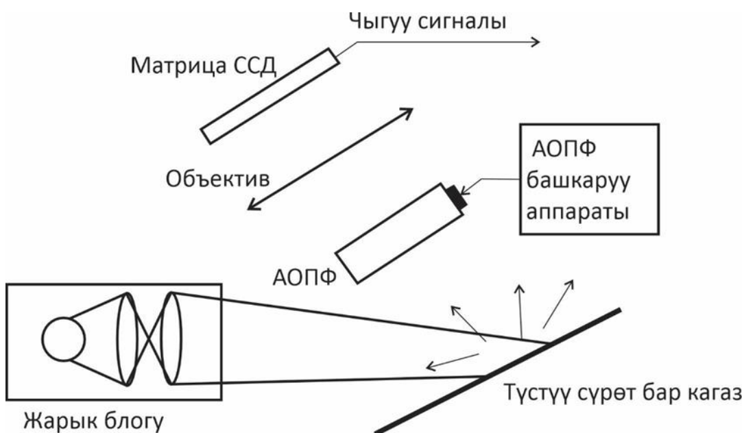
11-сүрөт. Кагаз фонунун оптикалык конфигурациясы жана АОПФ аркылуу символдордун спектралдык курамы.
