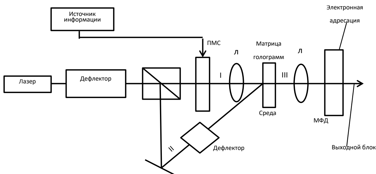
Рисунок 2.1. Блок-схема голографической памяти
