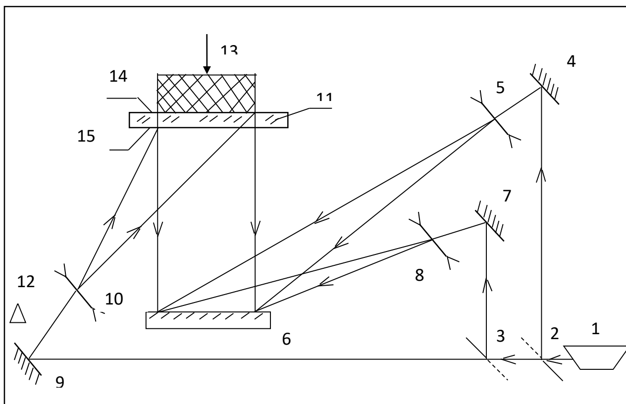
Рисунок 1.11. Схема устройства определения микро-перемещений в плоскостях.
