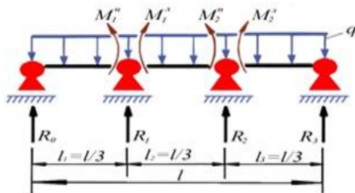
Рисунок 2.5.5 – Трёхпролётная схема.
