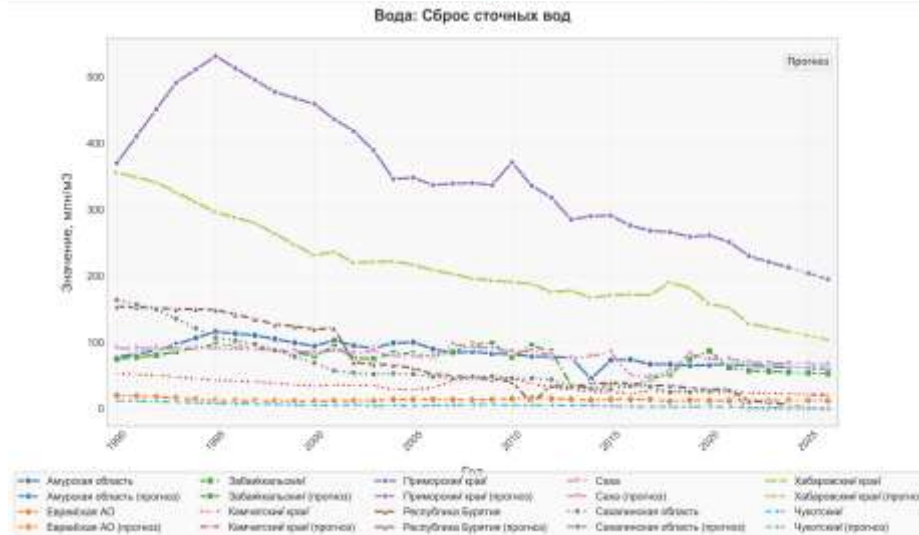
Рисунок 2.3. – Динамика сброса загрязненных сточных вод в поверхностные водные объекты УФО, СФО, ДФО, млн м³ (составлено автором)
