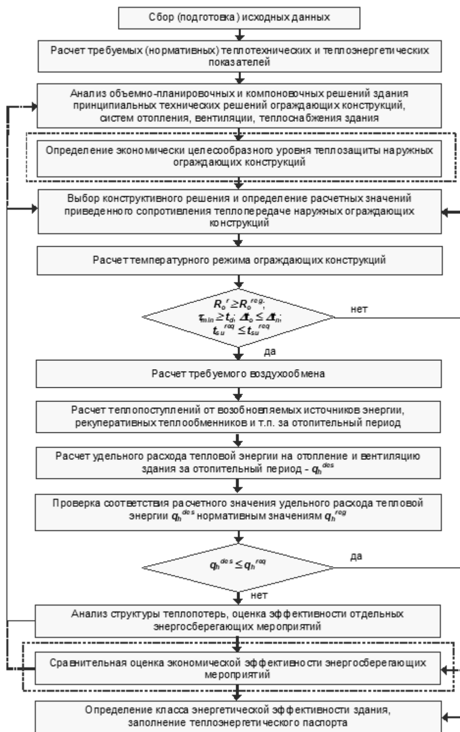
Рисунок 3.4 – Блок-схема алгоритма
